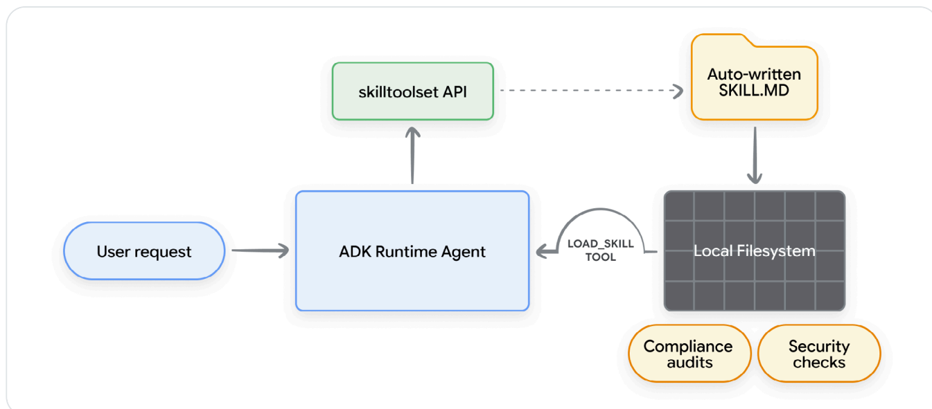
شکل ۹: این حلقه گام به گام نشان می‌دهد چگونه تاریخچه‌های واقعی و موفق تولید، بدون پیش‌نویس‌نویسی دستی انسان، به حافظه‌های روبه‌ای قابل‌اتکا بدل می‌شوند.
