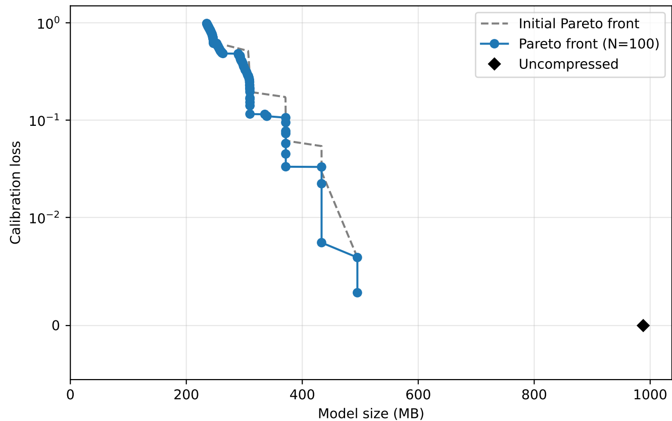
Generation 50 HV 0.3679
