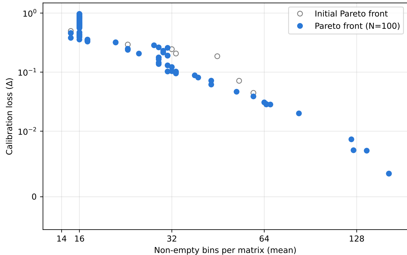
Generation 50 HV 0.1843
