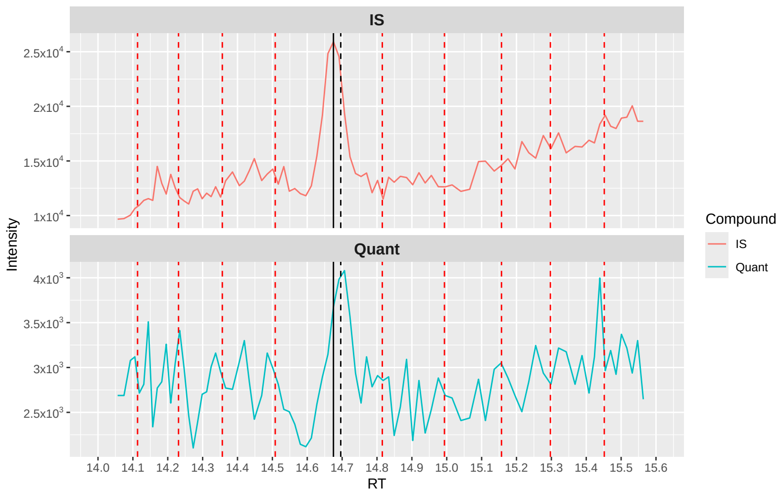
RvT4 Quant (m/z 361.1 → 211.1): Chow 2 (7500)
