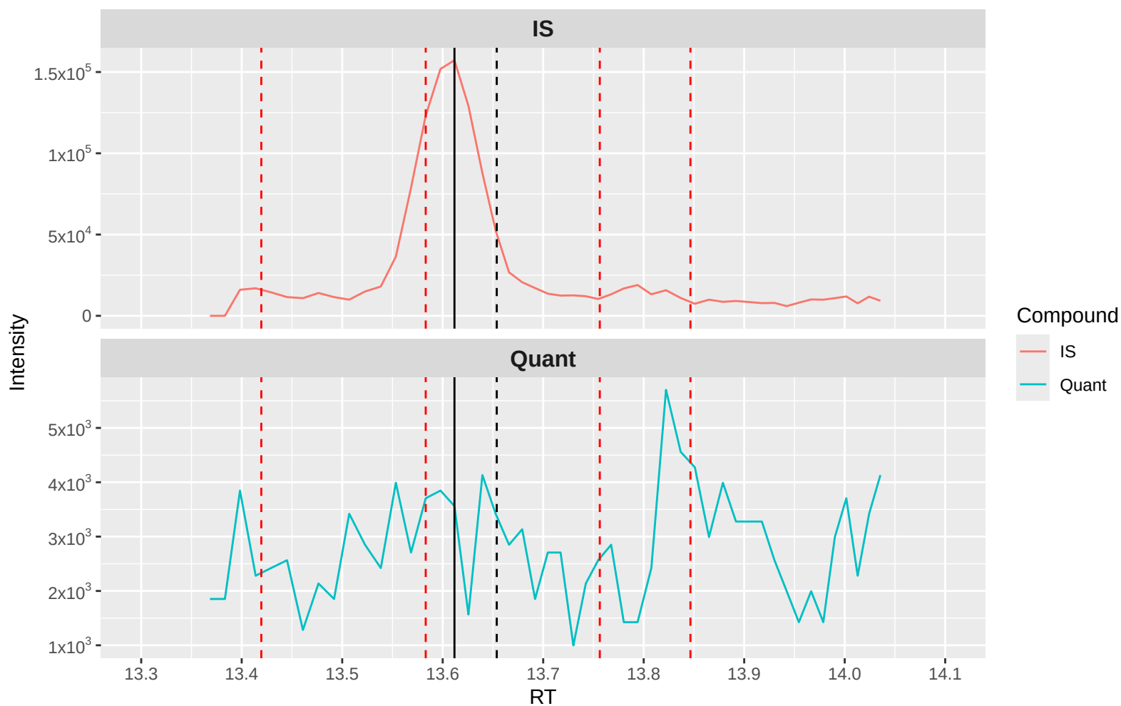
RvT4 Quant (m/z 361.1 → 211.1): Chow 4 (6500)
