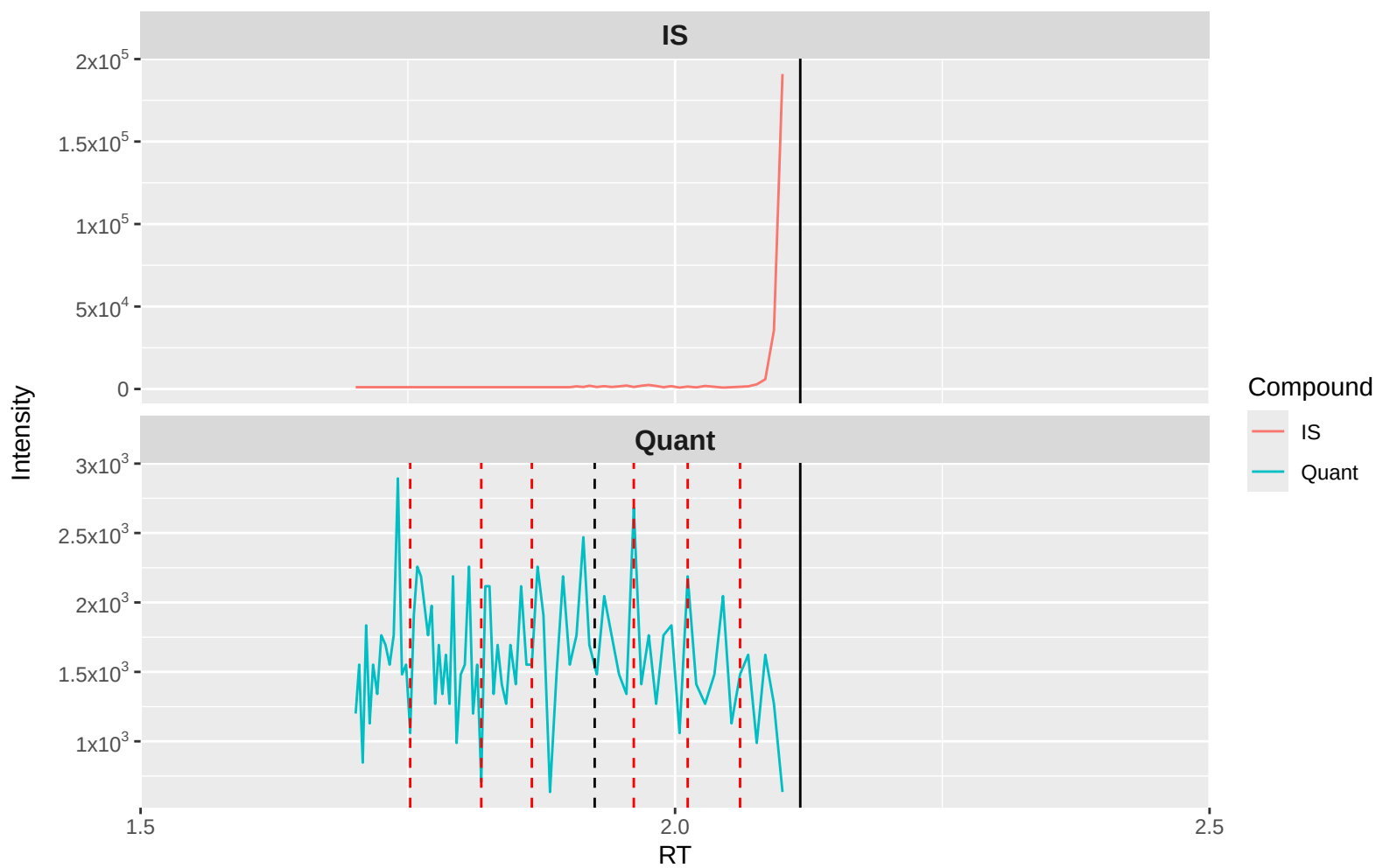
Ketamine Quant (m/z 238 → 125): ketamine inj 15 (sciex)
