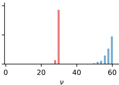
classical- t , p = 80
