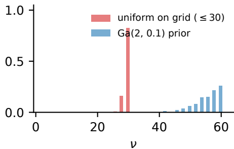
classical- t , p = 40
