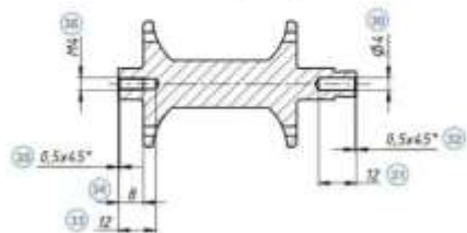
A-A (1:1)
