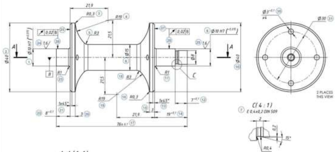
A-A (1:1)
