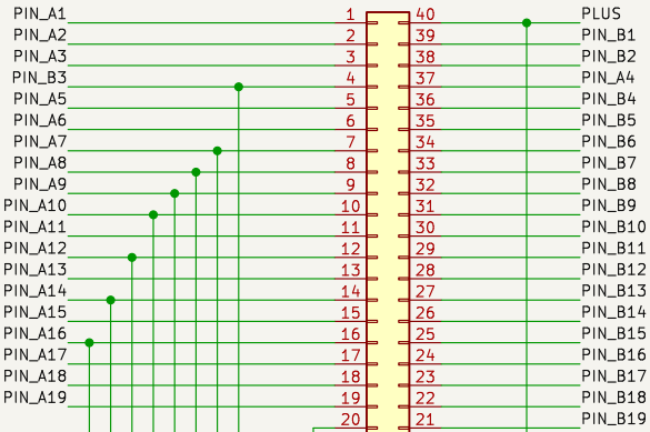
J1 ZIF Device Under Test
