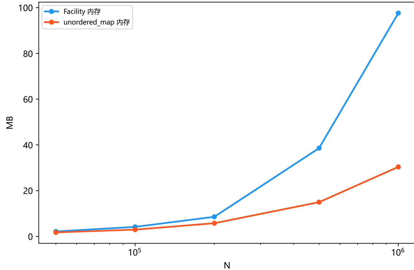
良好哈希
