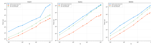
图 5-5 插入/查询/删除综合对比（对数-对数尺度）
