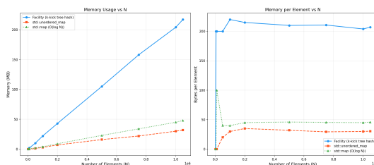
图 5-4 内存占用对比（总计 + 每元素）
