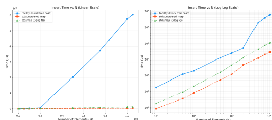
图 5-1 插入时间对比（线性 + 对数-对数尺度）
