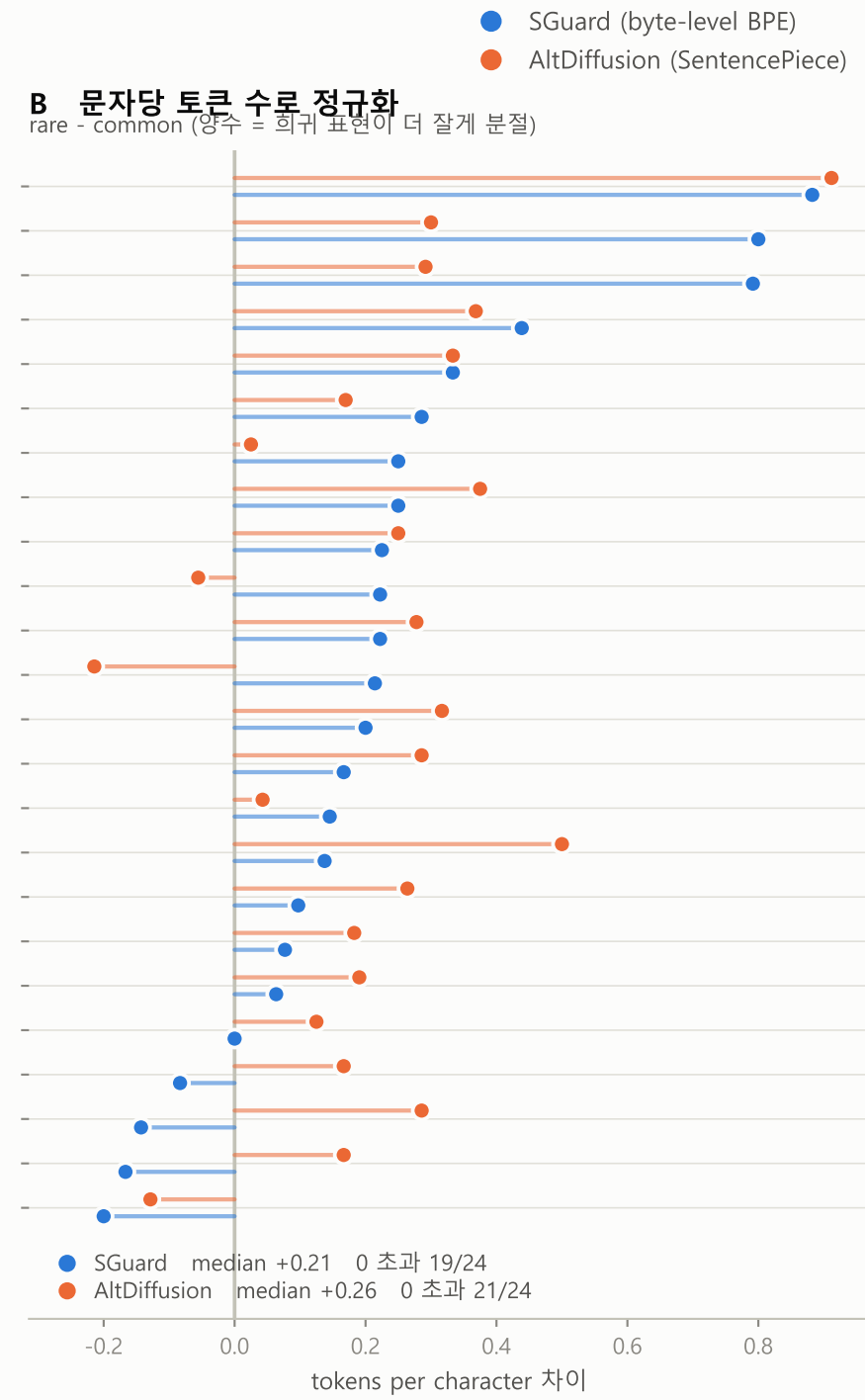
Figure A 희귀 한국어 표현의 토큰 분절 — 정규화 여부로 결론이 뒤집힌다 concept 24쌍 paired 비교. y축 라벨은 concept_id 와 rare 표현 (진한 라벨 = unsafe concept). 두 패널의 concept 순서는 동일하다.
