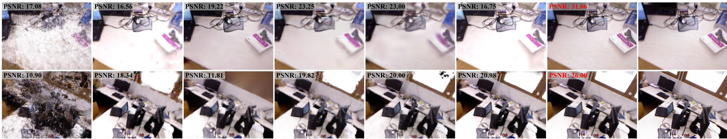
TUM RGB-D
