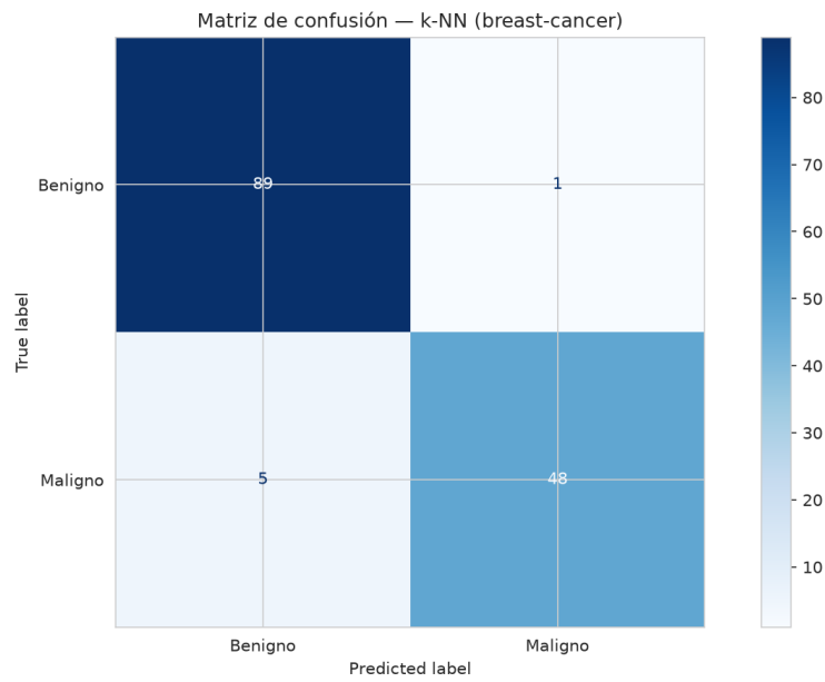
Figure 3: Matriz de confusión del clasificador k-NN (test).
