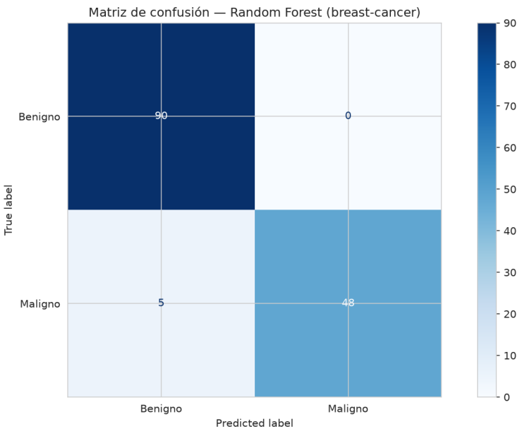
Figure 14: Matriz de confusión del Random Forest (test).
