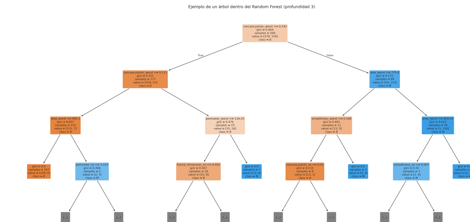
Figure 16: Ejemplo de un árbol dentro del bosque (profundidad 3) graficado con plot_tree .
