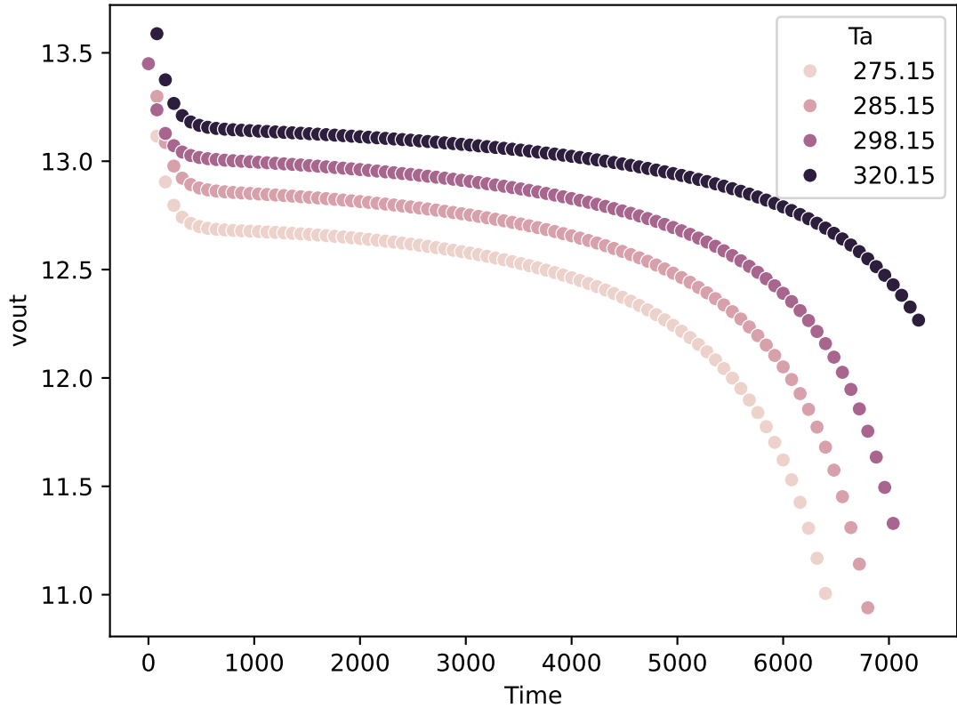
vout_over_time
