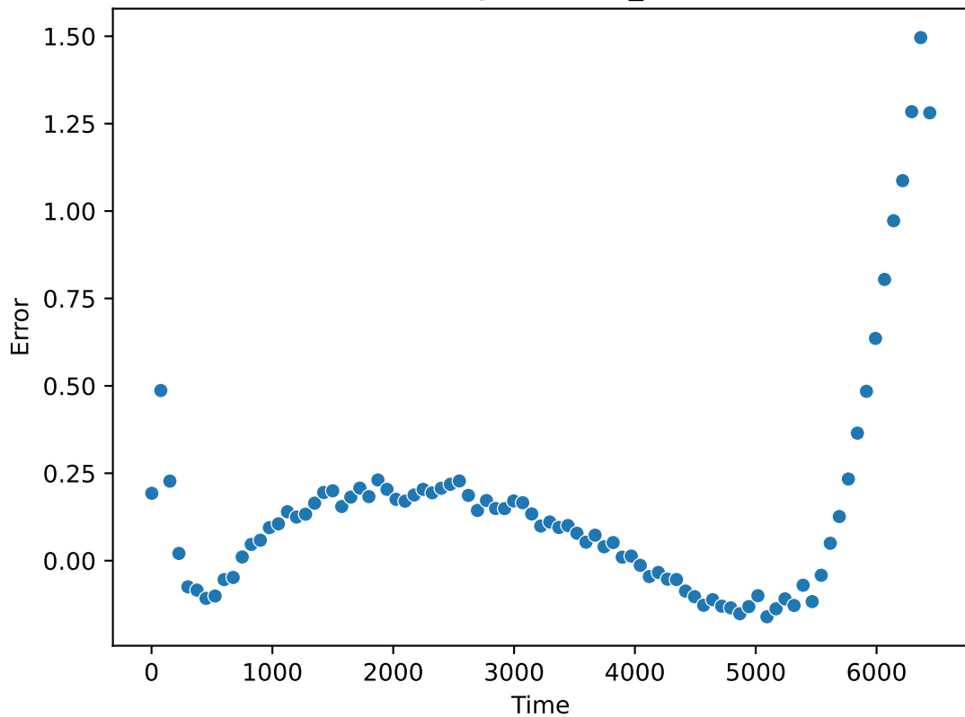
VoltageError-err_rel
