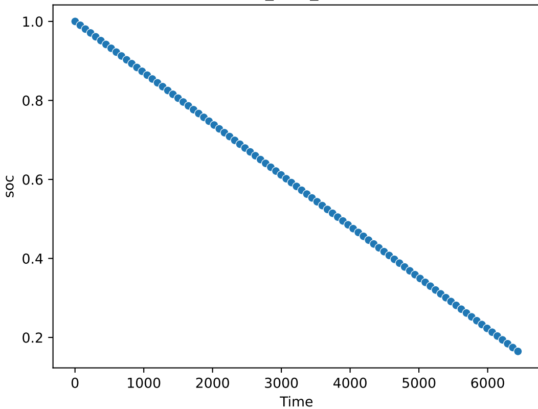
soc_over_time
