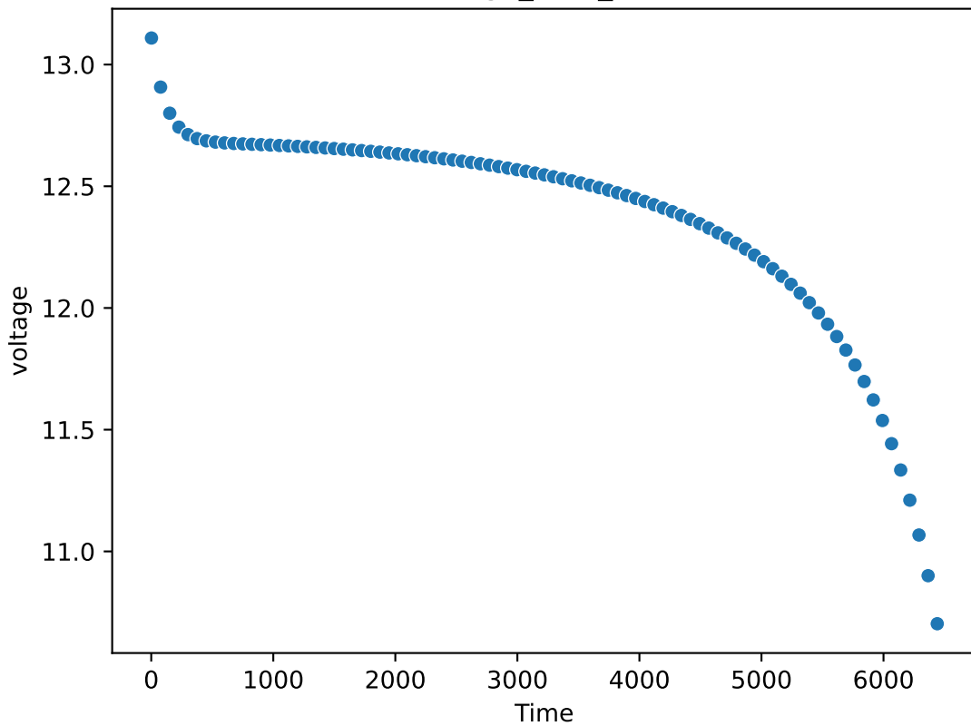
voltage_over_time
