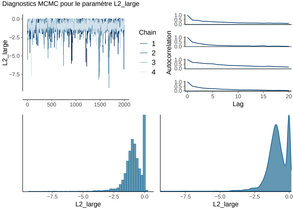
FIGURE 5.3 – Exemple de diagnostics MCMC illustrés pour le paramètre L2_large, sélectionné à partir du modèle global. De gauche à droite et de haut en bas : (1) traceplot des chaînes, un bon mélange est souhaité et se traduit par des chaînes entrelacées, similaires à un bruit blanc ; (2) fonction d’autocorrélation, une décroissance rapide vers zéro est souhaitée, ce indique une faible dépendance entre échantillons successifs ; (3) histogramme de la distribution a posteriori , il doit contenir assez d’informations pour approximer la densité ; (4) courbe de densité estimée a posteriori , l’axe x de l’histogramme et de la courbe de densité est exprimé en taille d’effet standardisée.
