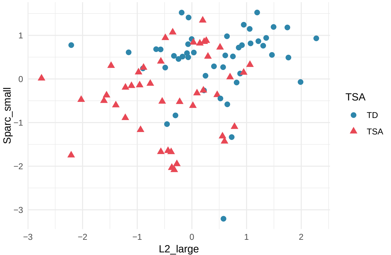
FIGURE 5.8 – Représentation des observations dans l'espace des deux variables sélectionnées par projection prédictive sur la tâche PA ( L2_large et Sparc_small ). Les unités des axes sont en taille d'effet standardisée.
