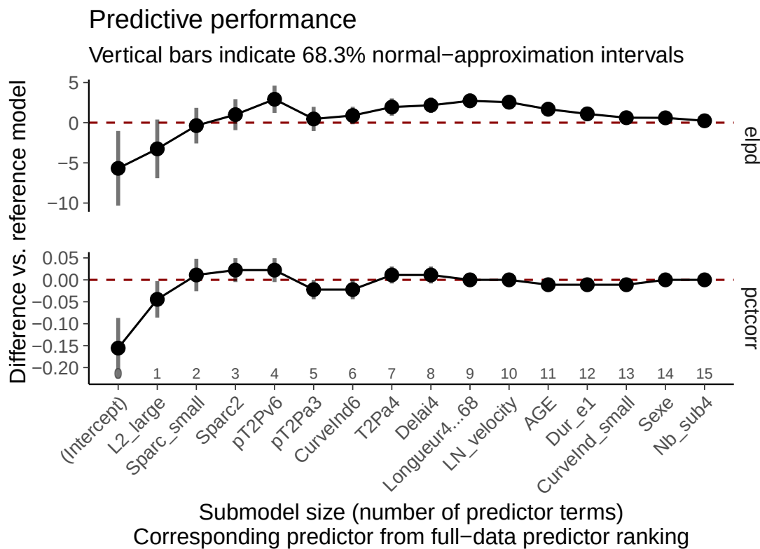
FIGURE 5.1 – Courbes de l'elpd et de l'accuracy issues du modèle de référence global, en fonction du nombre de variables incluses dans le sous-modèle, obtenues par projection prédictive avec validation croisée. Chaque point représente la différence d'elpd/d'accuracy entre le sous-modèle et le modèle de référence. Les barres d'erreur indiquent l'incertitude à \pm 1 erreur standard. Une différence proche de zéro indique des performances prédictives équivalentes au modèle de référence global.
