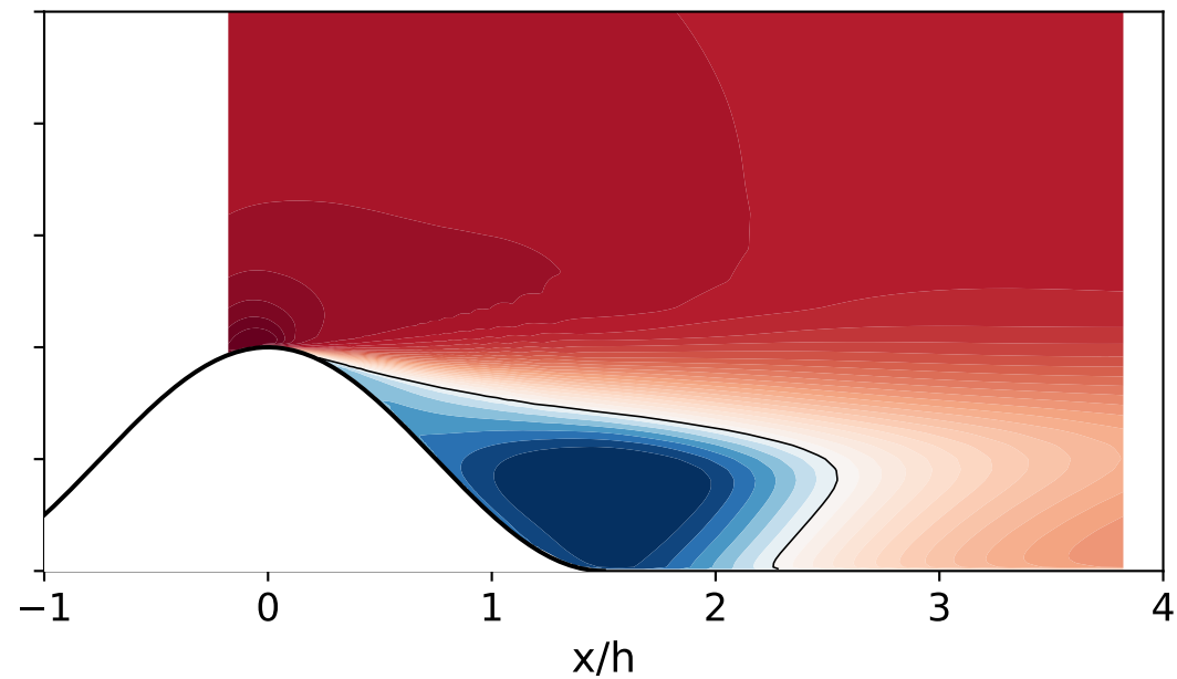
Baseline k- \omega SST
