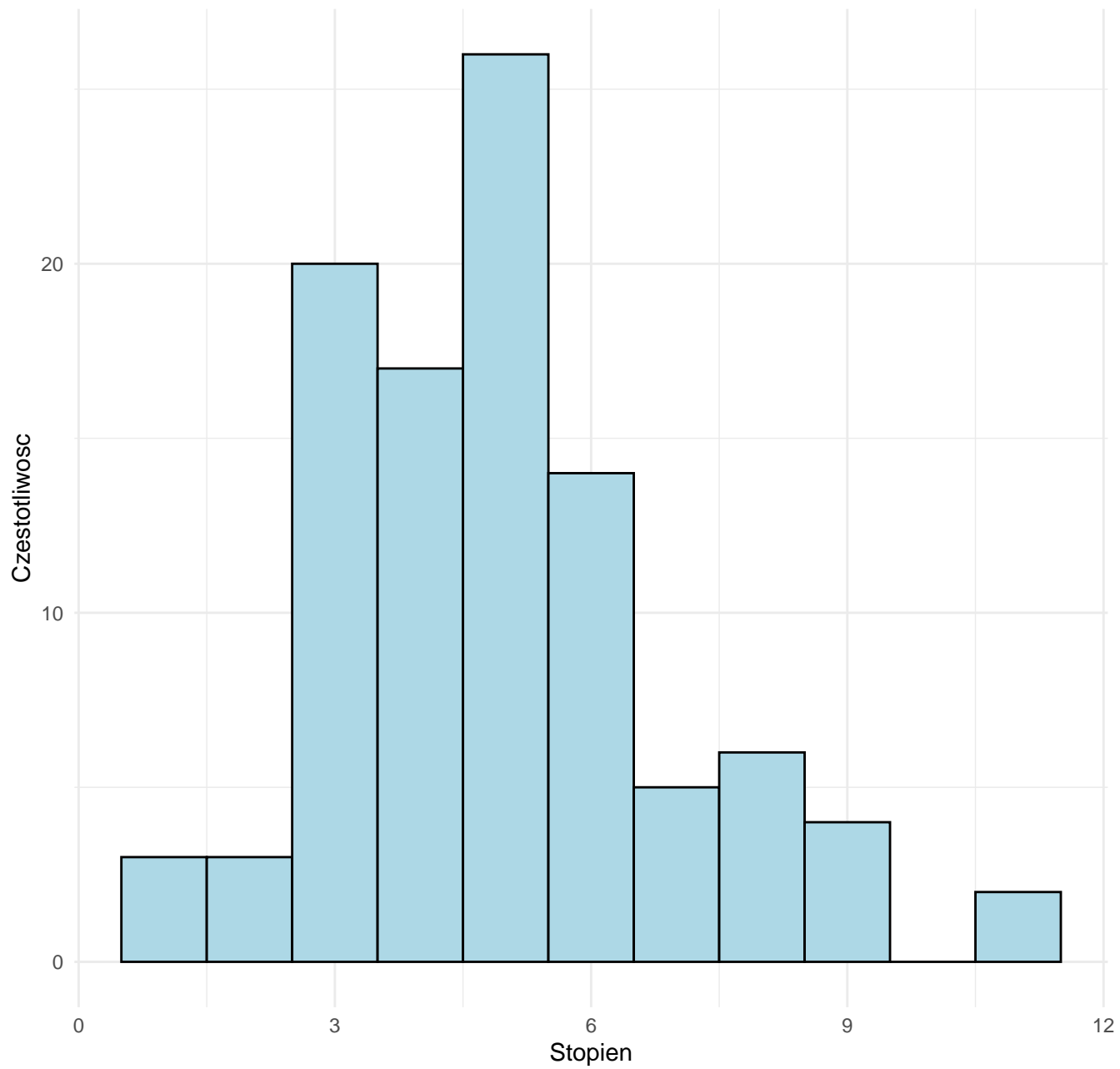
Histogram stopni wezlow
