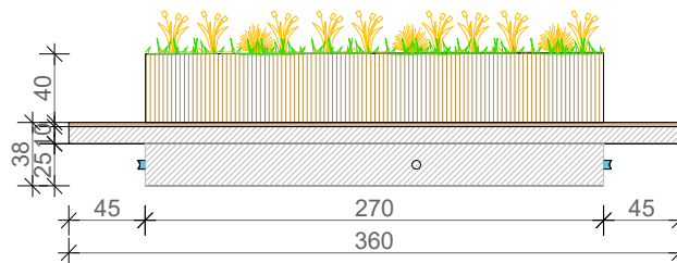
ПРЕСЕК 2-2
