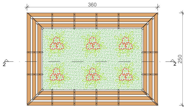
ИЗГЛЕД
