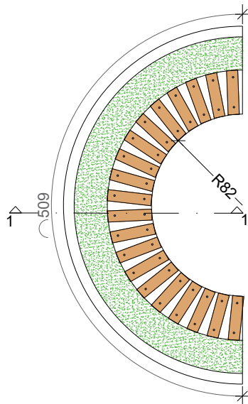
ПРЕСЕК 1-1
