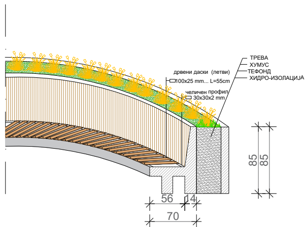
ПРЕСЕК 1-1
