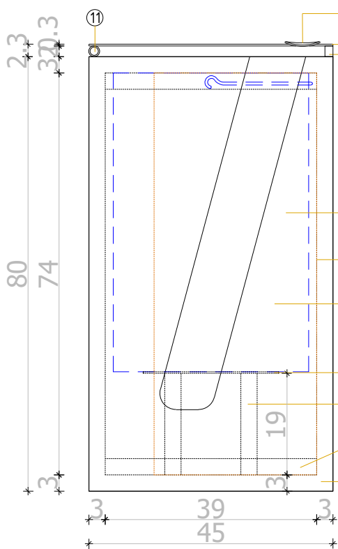
ПРЕДЕН ИЗГЛЕД
