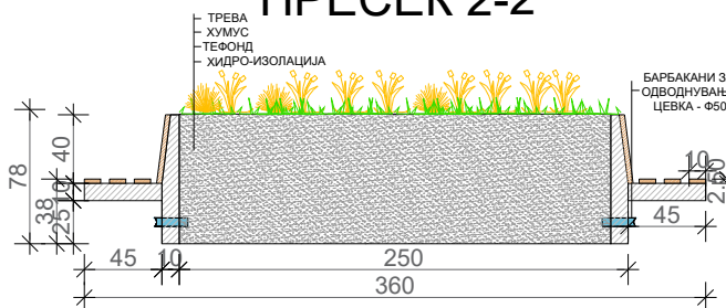
ПРЕСЕК 2-2
