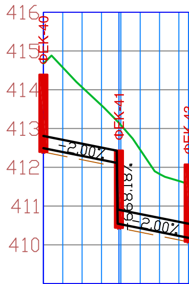
DN200 PPHM L=37.51m
