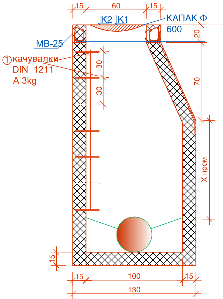
ПРЕСЕК 2-2
