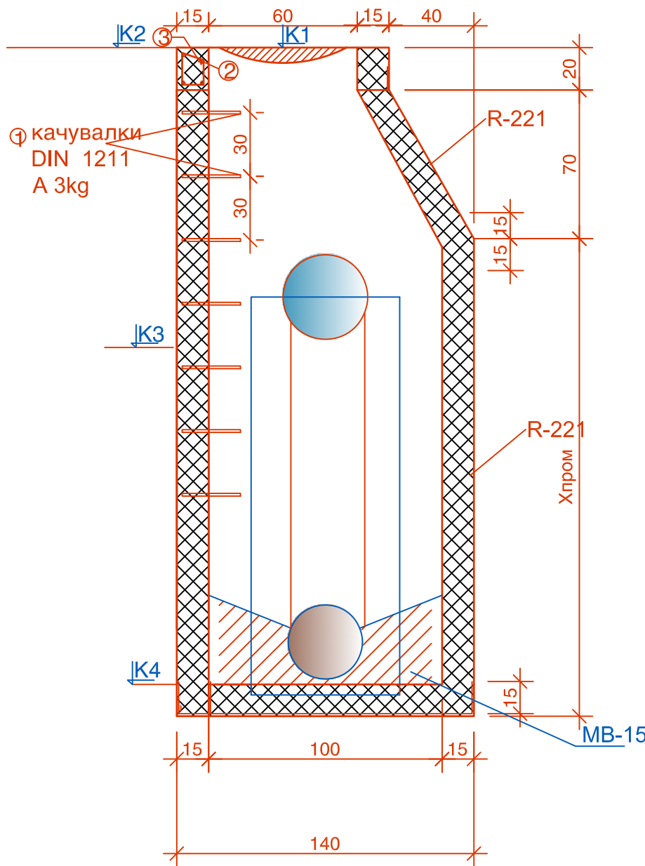
ПРЕСЕК 2-2
