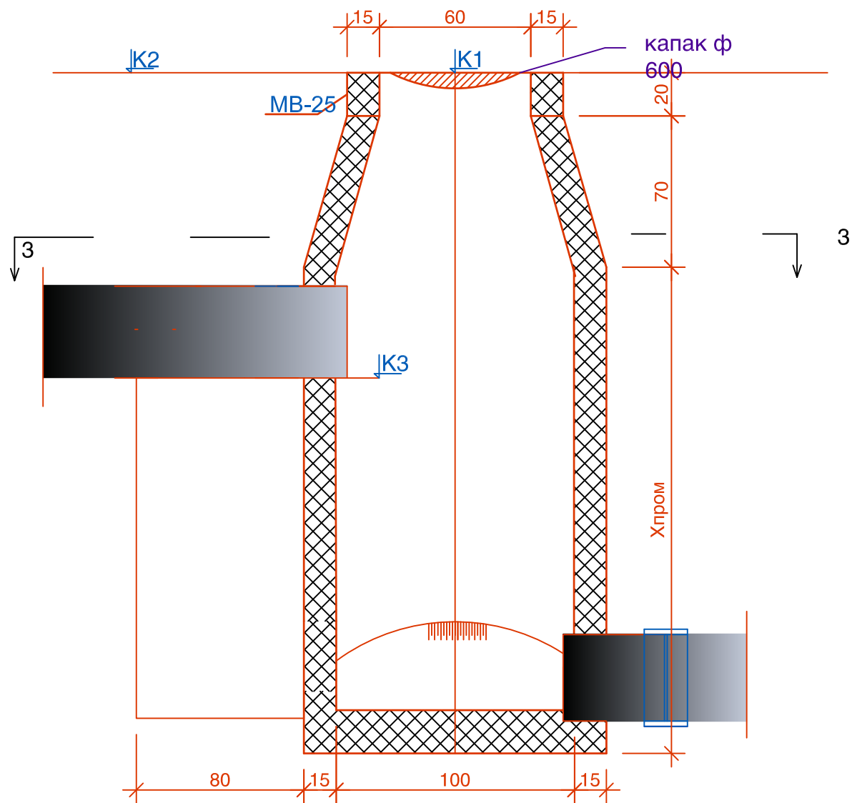
ПРЕСЕК 1-1
