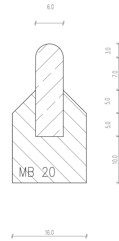
РАБНИК ТИП ПАВЕР 6/20/100 М = 1:10 (sm)
