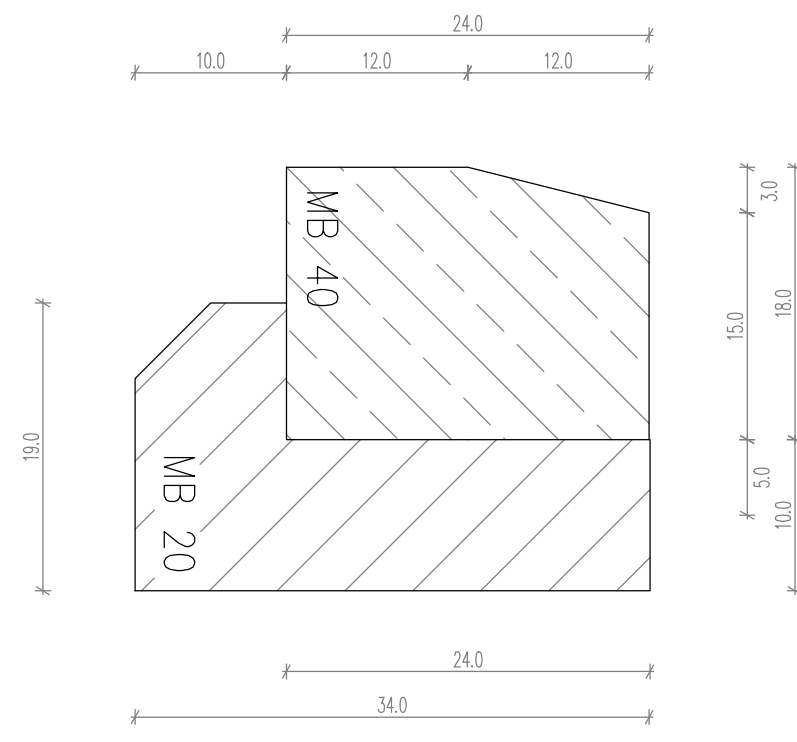
БЕТОНСКИ РАБНИК 18/24 МВ-40 М = 1:10 (sm)
