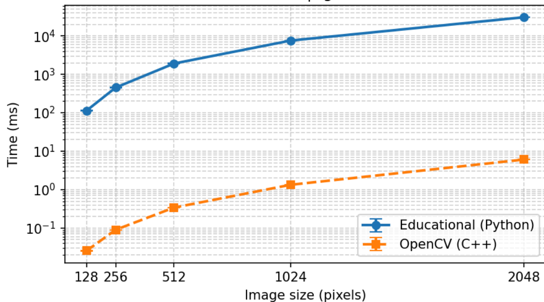
blur_3x3 zero | rgb
