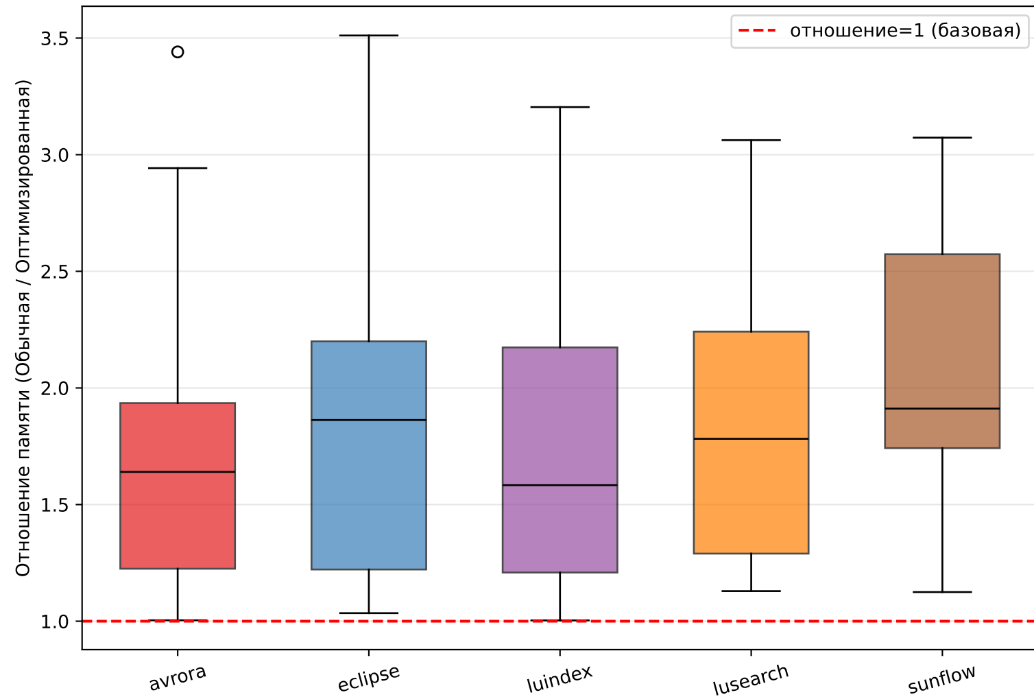
Сокращение памяти по графам (>1 означает, что оптимизированная использует меньше)
