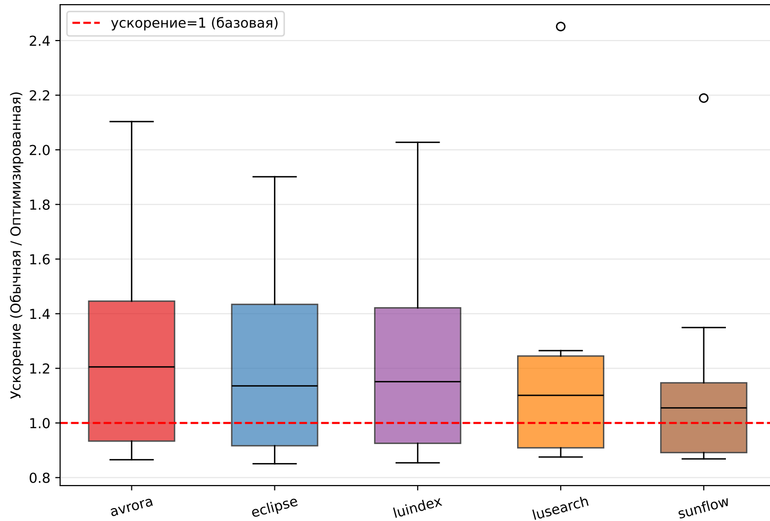
Ускорение по графам (>1 означает, что оптимизированная быстрее)
