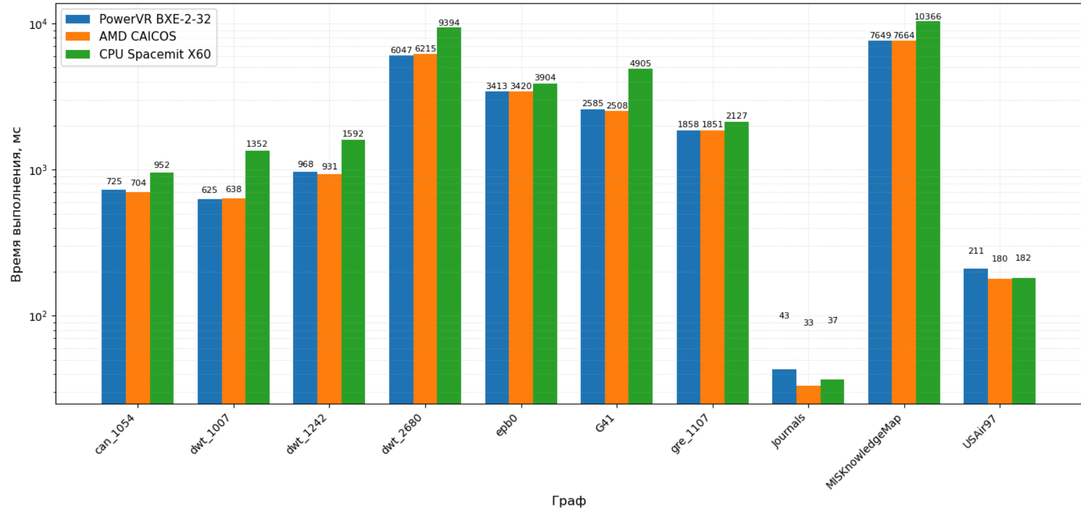
Сравнение производительности SpIa на трёх платформах
