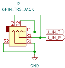
Input Jack
