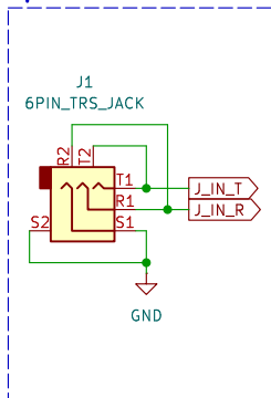
Input Jack
