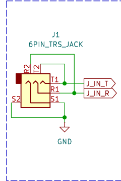
Input Jack
