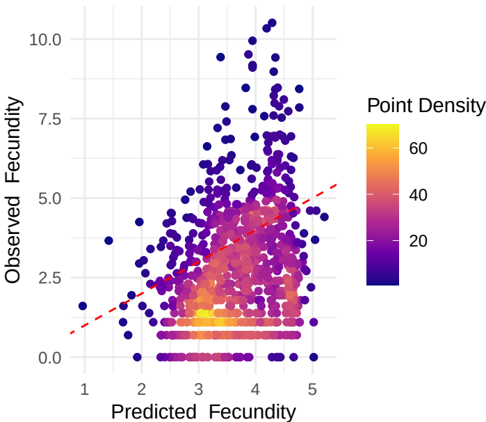
F Testing Posterior
