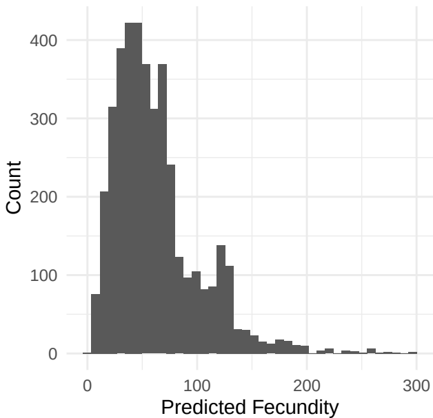
F Testing Posterior
