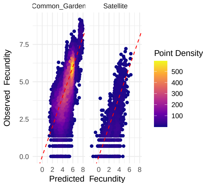
Training Posterior
