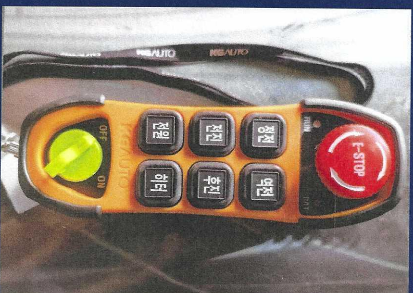
무선조작리모콘
