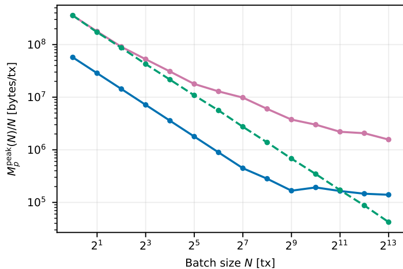
(d) Mean peak memory per transaction
