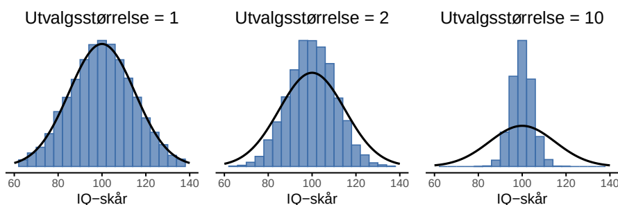
(a) Fordelingen til gjennom(b) Fordelingen til gjen(c) Fordelingen til gjennom- snittene er den samme somnsnittene er smalere ennnsnittene er mye smalere enn fordelingen til populasjonenfordelingen til populasjonenfordelingen til populasjonen
