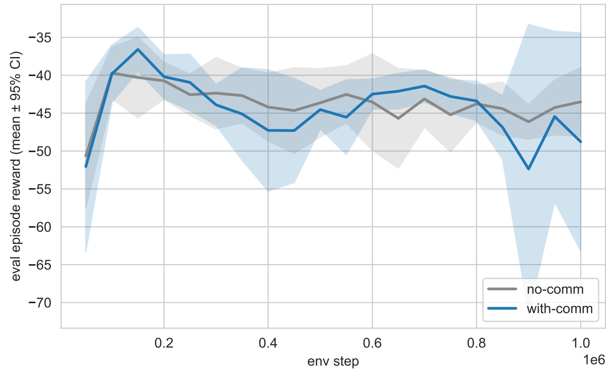
IQL
