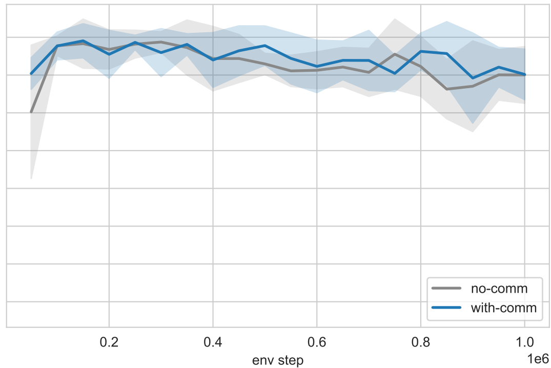
VDN
