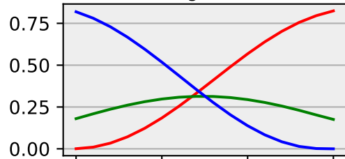
posterior geodesic
