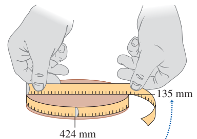
Figura 1.8 Como determinar o valor de \pi a partir da circunferência e diâmetro de um círculo.
