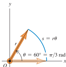
Figura 9.11 Sempre use radianos ao relacionar grandezas lineares com grandezas angulares.
