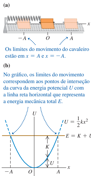
Figura 7.23 (a) Um cavaleiro sobre um trilho de ar. A mola exerce uma força F_x = -kx . (b) A função da energia potencial.
