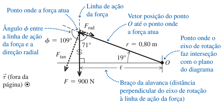
(b) Diagrama de corpo livre
