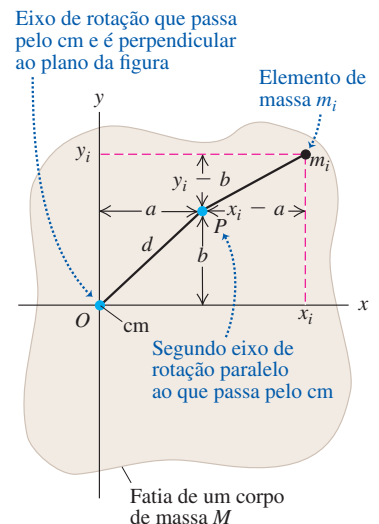
Figura 9.20 O elemento de massa m_i possui coordenadas (x_i, y_i) em relação ao eixo que passa no centro de massa (cm) e coordenadas (x_i - a, y_i - b) em relação ao eixo paralelo que passa no ponto P .
