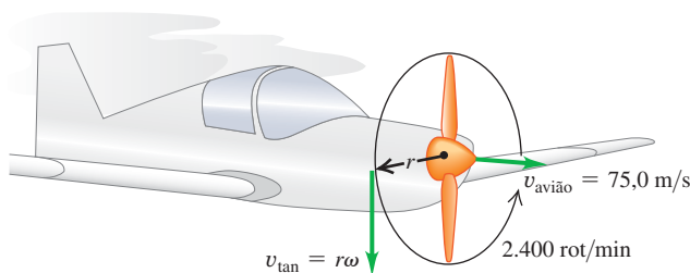
Figura 9.13 (a) Um avião com propulsão a hélice em voo. (b) O esquema indica os componentes de velocidade para a extremidade da hélice.
