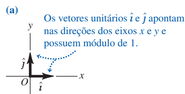
Figura 1.24 (a) Os vetores unitários \hat{i} e \hat{j} . (b) Podemos expressar um vetor \vec{A} em termos dos seus componentes.
