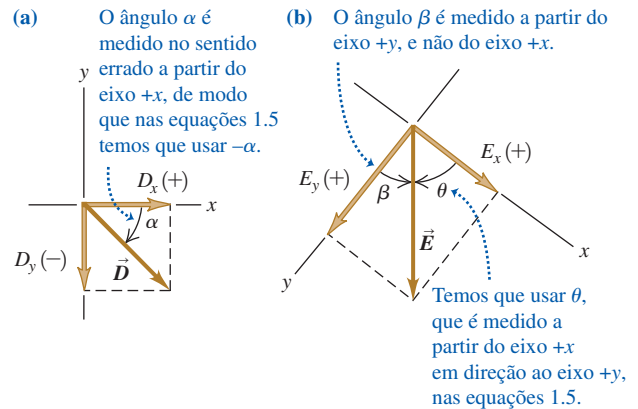
Figura 1.19 Cálculo dos componentes x e y de vetores.
