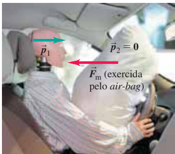
Figura 8.4 O teorema do impulso-momento linear explica como os air-bags reduzem a possibilidade de lesões minimizando a força sobre o ocupante de um automóvel.
