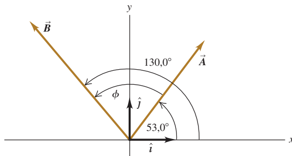
Figura 1.28 Dois vetores \vec{A} e \vec{B} em duas dimensões.
