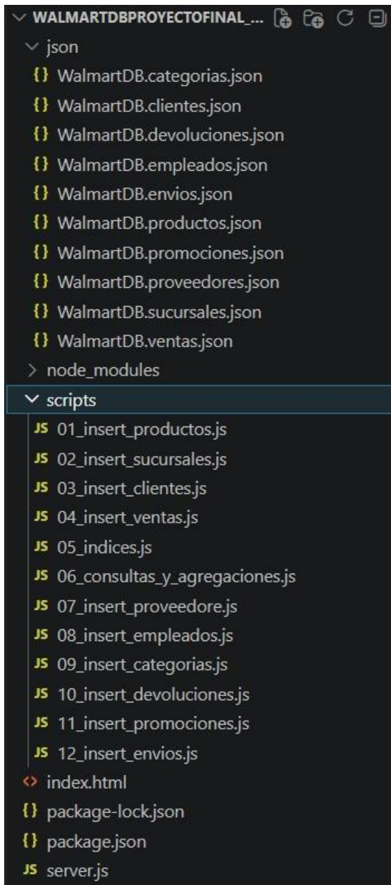
Figura 1. Estructura general del proyecto desarrollada en Visual Studio Code. En ella se observa la organización de los archivos JSON utilizados como fuente de datos y los scripts empleados para la inserción, consulta y administración de la base de datos.
