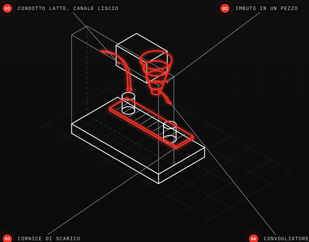
FIG. 01 - VISTA ISOMETRICA
