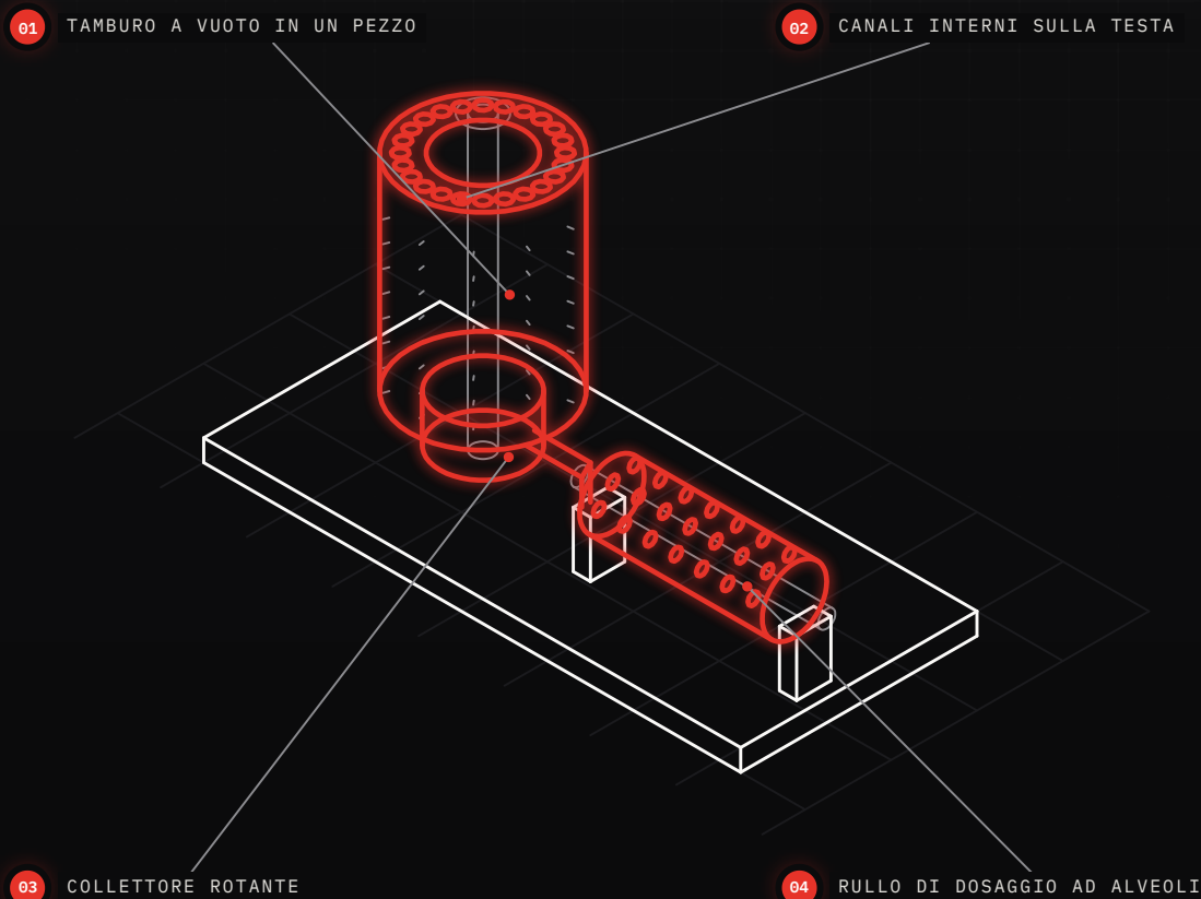
FIG. 01 - VISTA ISOMETRICA
