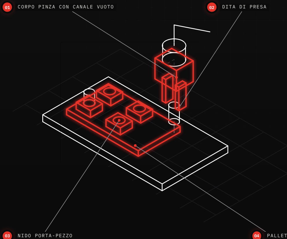
FIG. 01 - VISTA ISOMETRICA
