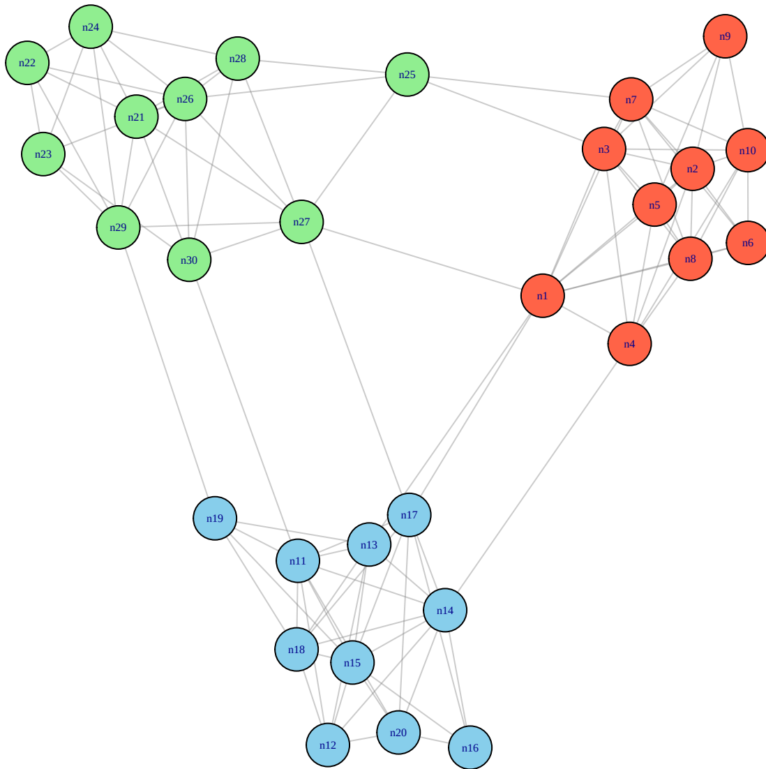
Figure 7.2: Ejemplo visual: red con 3 comunidades claramente separadas
