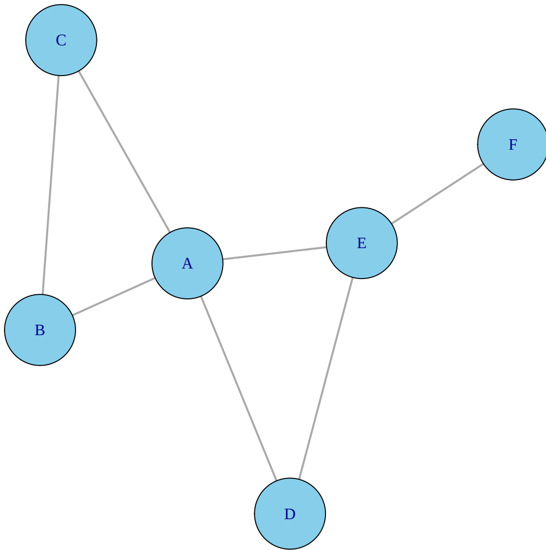
Figure 4.3: Red de ejemplo para calcular clustering local
