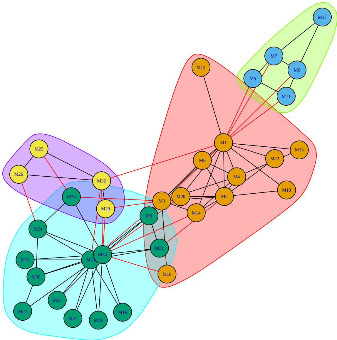
Figure 7.7: Comunidades por Louvain
