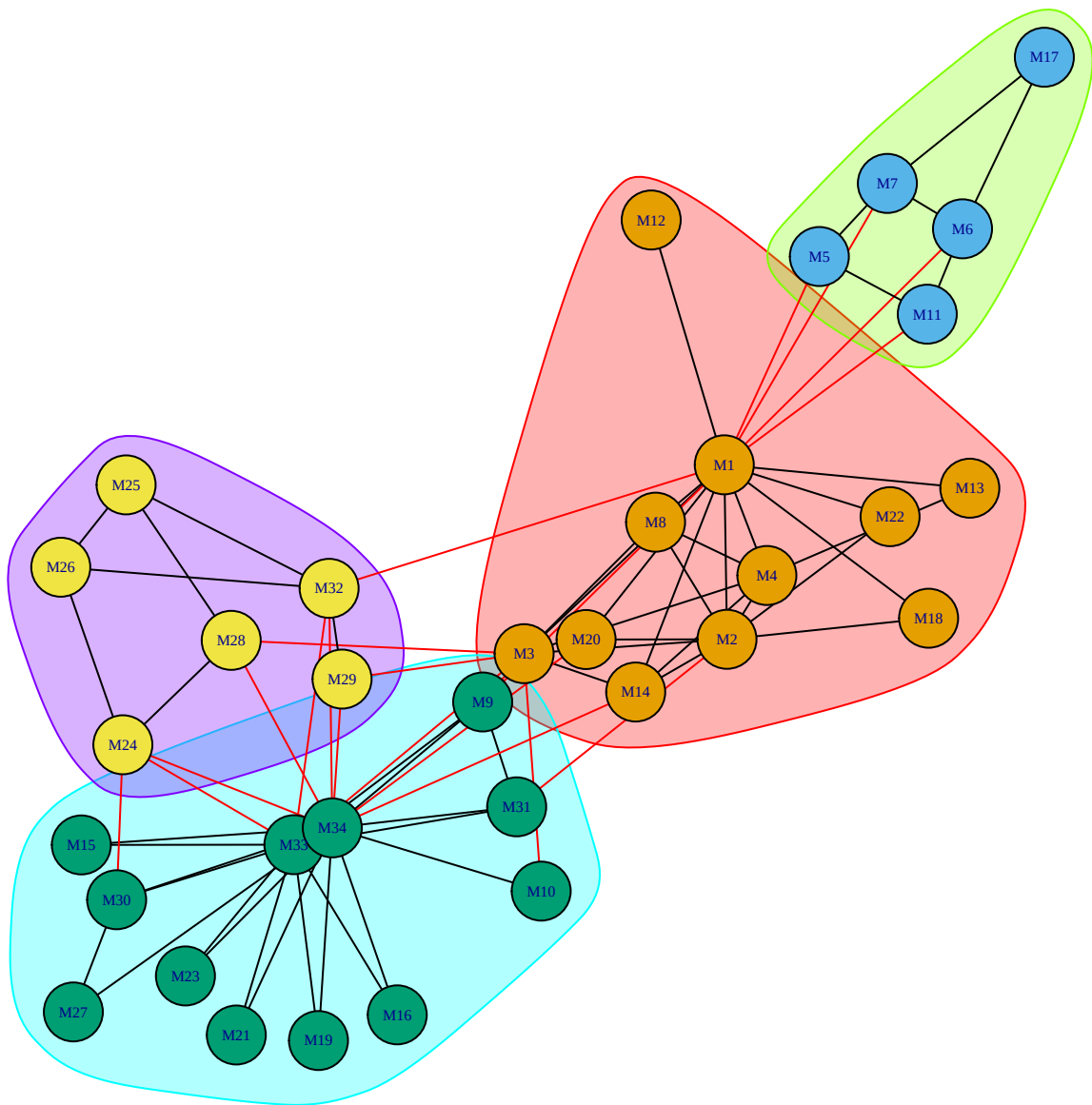
Figure 7.13: Comunidades por optimización exacta de modularidad
