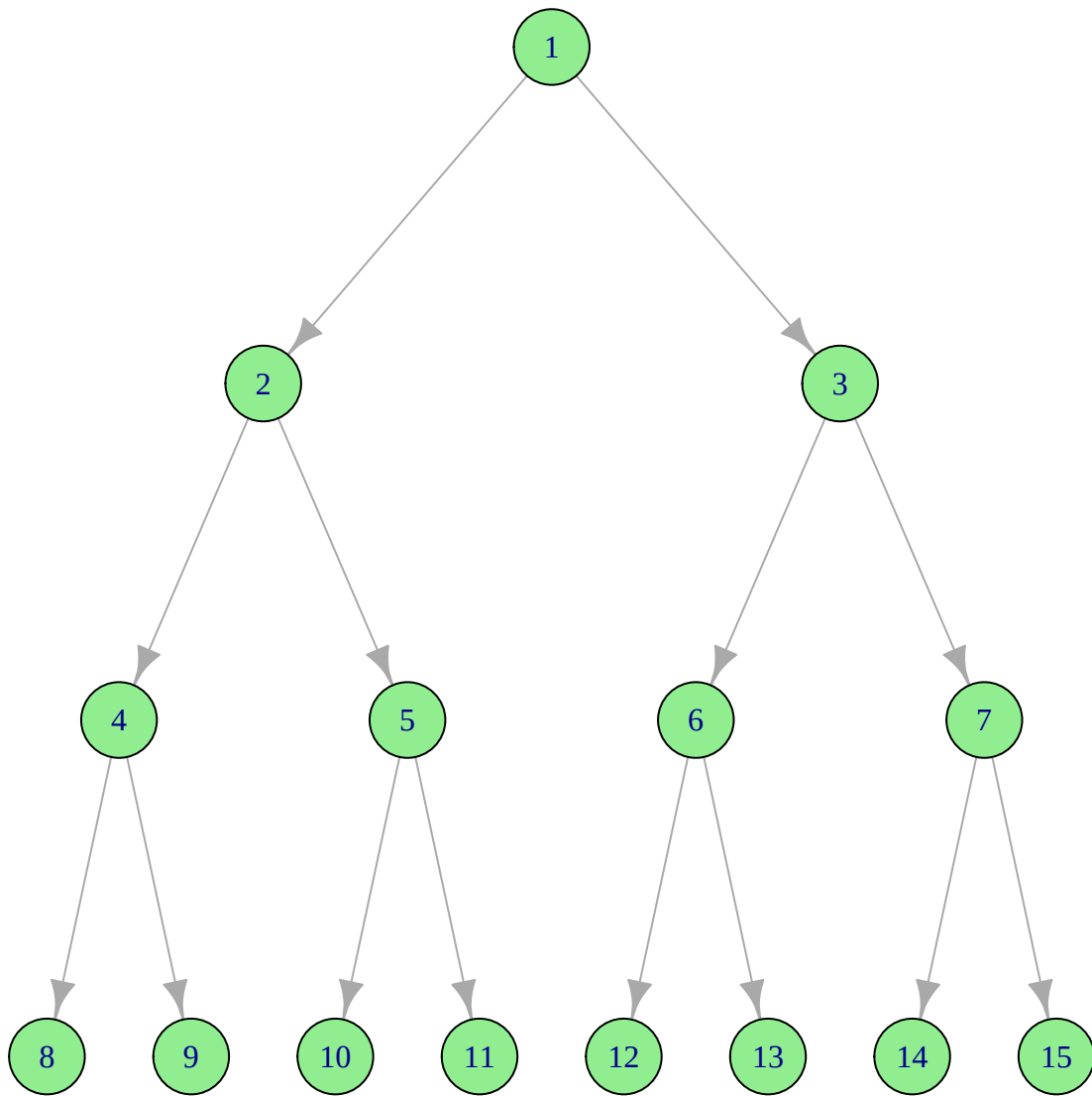
Figure 1.10: Árbol binario con 15 nodos
