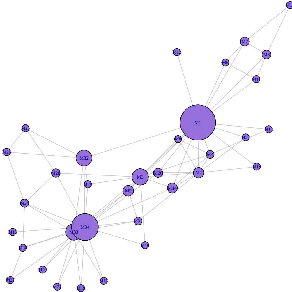
Figure 6.5: Red con nodos escalados por centralidad de intermediación
