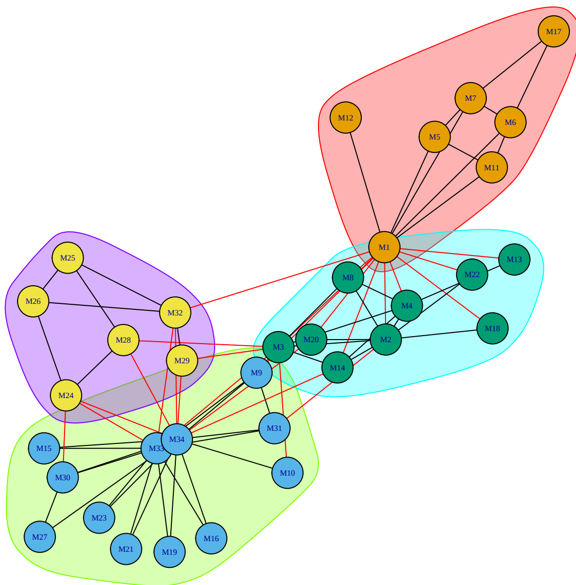
Figure 7.6: Comunidades por leading eigenvector
