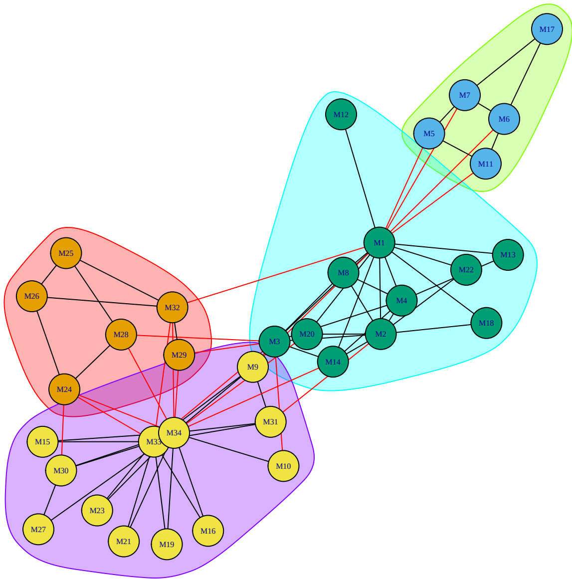
Figure 7.10: Comunidades por spinglass
