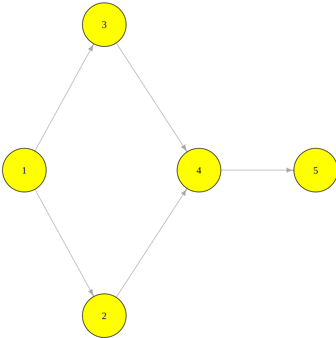
Figure 1.3: Red con conexiones agregadas manualmente
