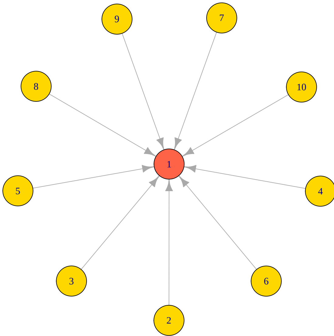
Figure 1.8: Red tipo estrella con 10 nodos
