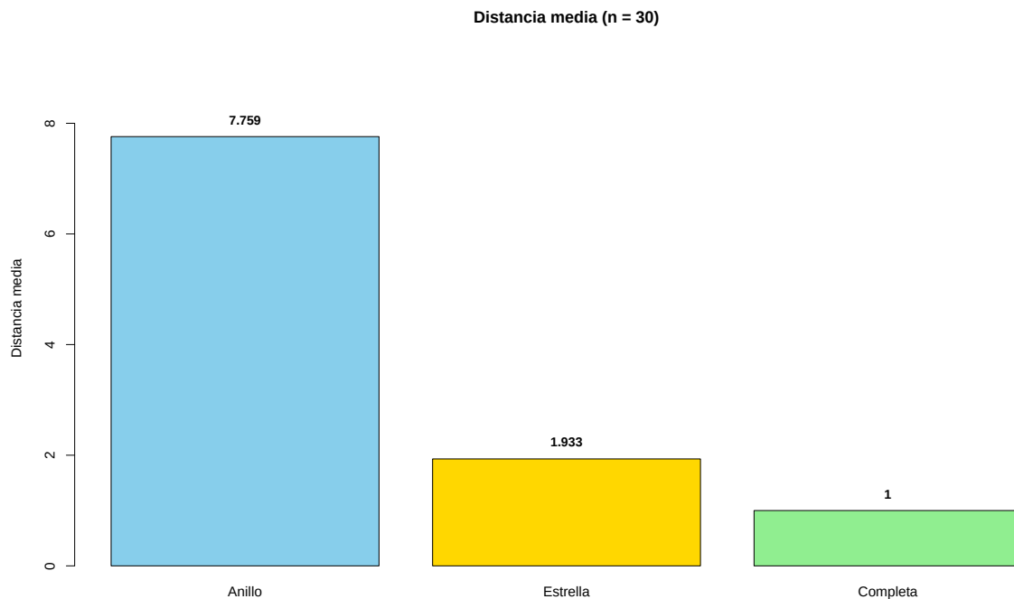
Figure 3.11: Distancia media de tres topologías con 30 nodos
