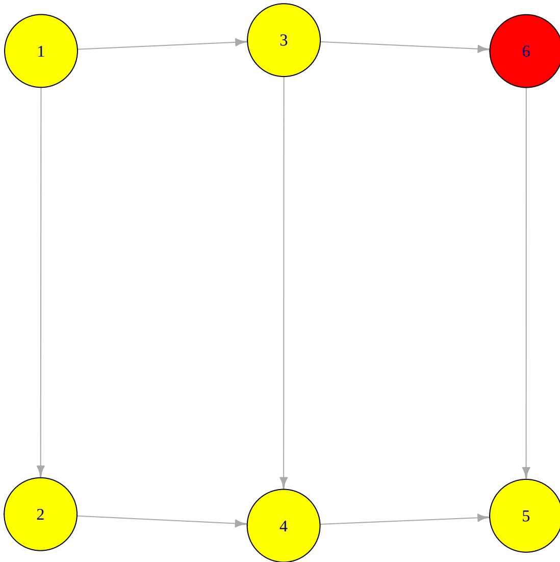
Figure 1.4: Nodo rojo agregado con nuevas conexiones
