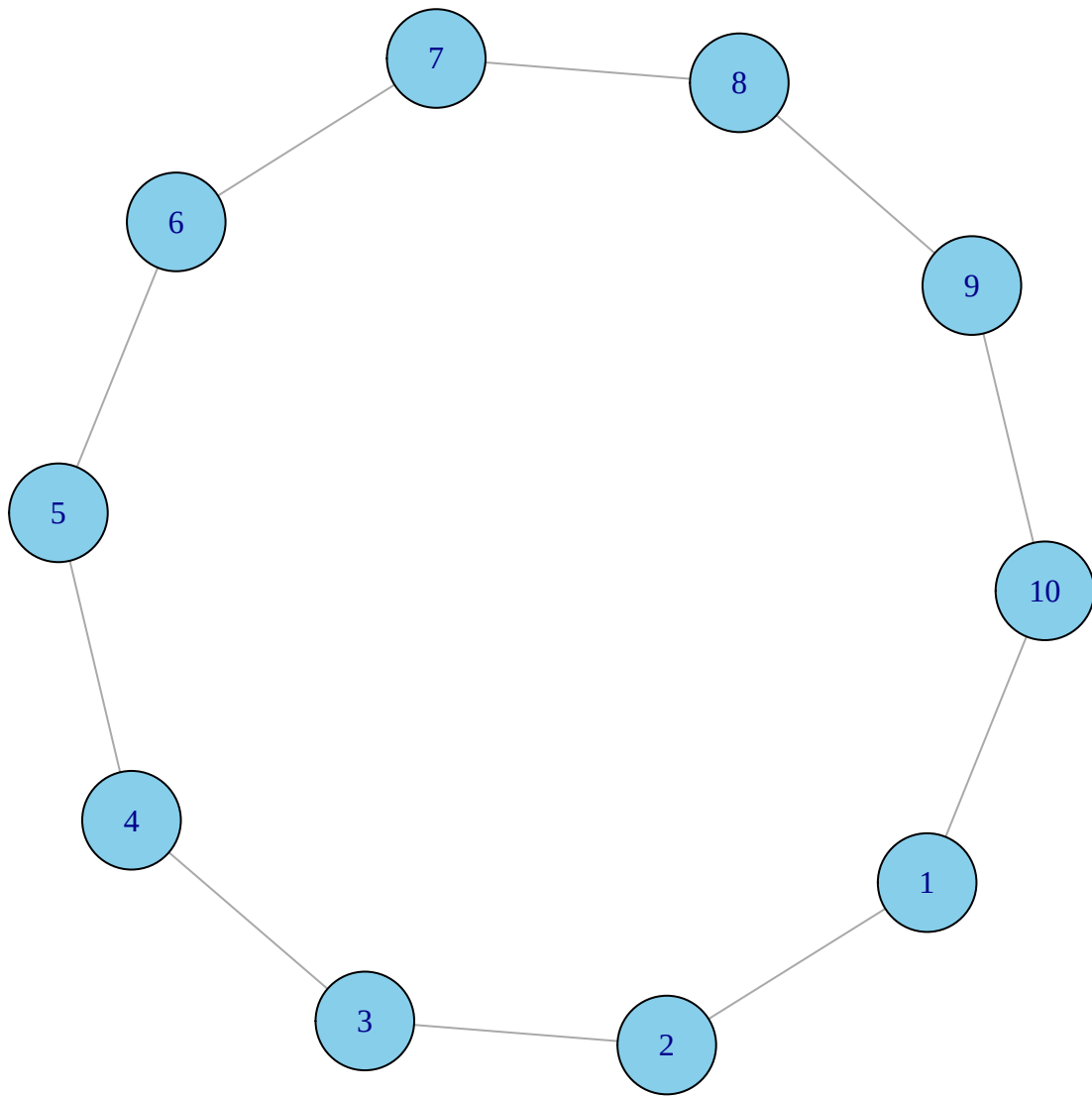
Figure 1.9: Red tipo anillo con 10 nodos
