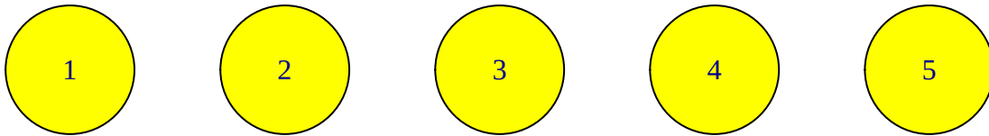
Figure 1.2: Red vacía con 5 nodos y sin conexiones
