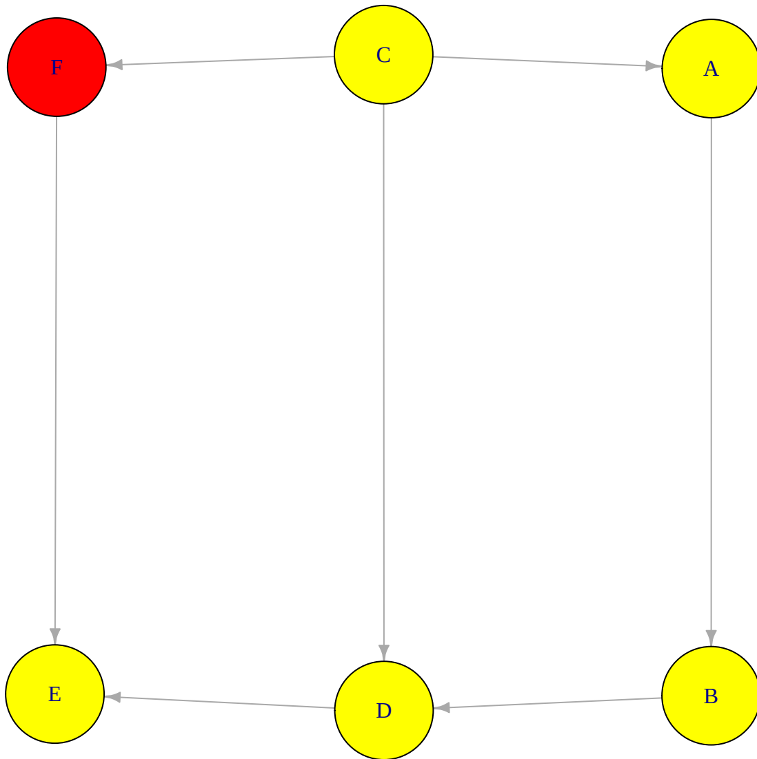
Figure 1.6: Red con dirección de conexión modificada
