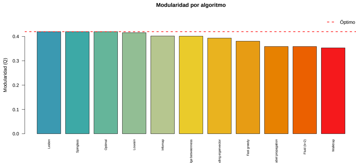
Figure 7.15: Modularidad de cada algoritmo en la red de Zachary
