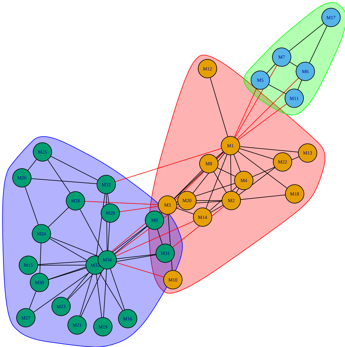
Figure 7.11: Comunidades por Infomap
