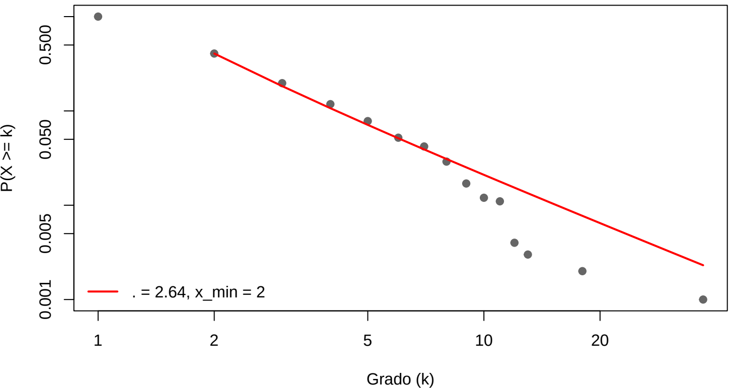
Ajuste Power-law - BA (n=1000)
