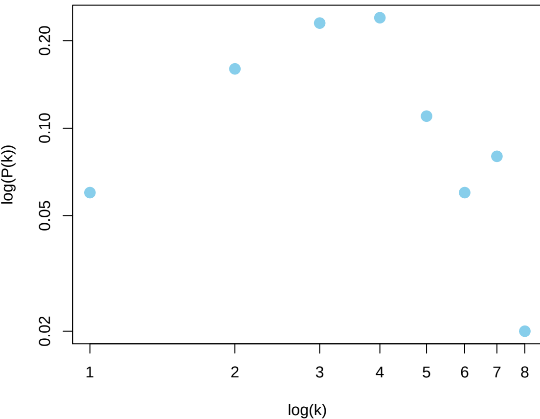
Log-log - Red ER
