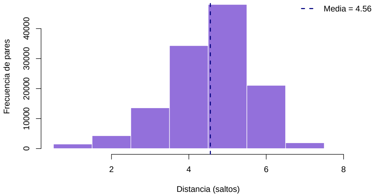
Figure 3.10: Distribución de todas las distancias en la red small-world de 500 nodos
