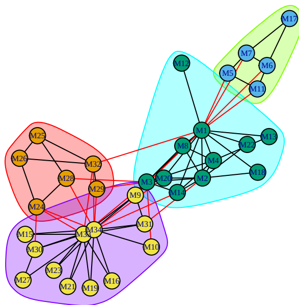
Figure 7.10: Comunidades por spinglass
