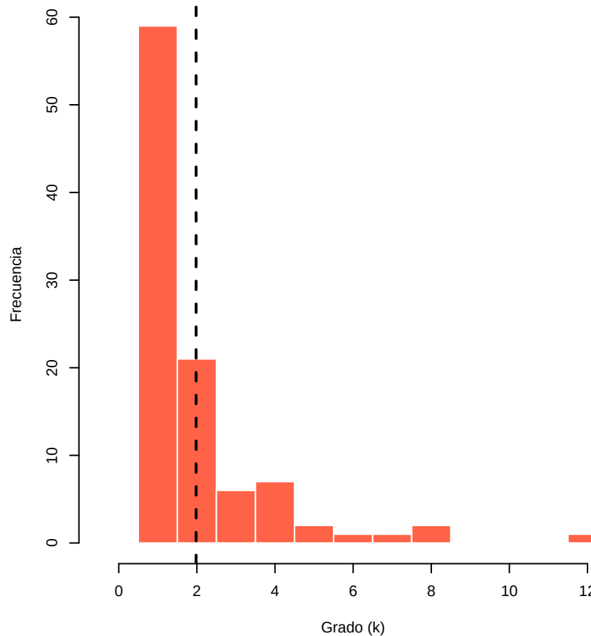
Barabási-Albert
