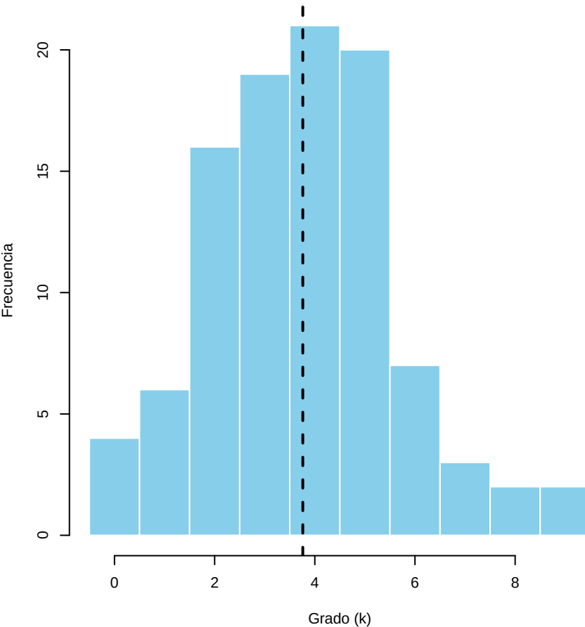
Erdős-Rényi
