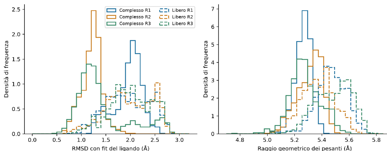
Figura 15.14A. Distribuzioni conformazionali nelle tre repliche del complesso 09k (linee continue) e nelle tre repliche del ligando libero 09j (linee tratteggiate), tutte da 10 ns. I colori identificano il numero della replica, senza implicare un accoppiamento statistico tra condizioni. RMSD con fit del ligando e raggio geometrico sono calcolati sui pesanti dopo lo scarto del primo 20%. Sono usati intervalli comuni per ciascun istogramma. Le deviazioni tra repliche richiedono una lettura separata e non dimostrano differenze di affinità.
