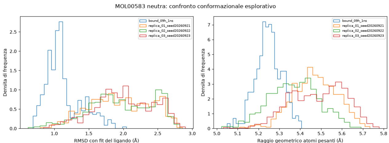
Figura 15.13A. Confronto preliminare tra MOL00583 libera in acqua (tre repliche 09j da 10 ns) e nel complesso della simulazione 09h da 1 ns. A sinistra, distribuzione dell'RMSD con fit del ligando rispetto a 09f; a destra, raggio geometrico degli atomi pesanti. È escluso il primo 20% di ciascuna produzione. Le finestre di campionamento differiscono: gli istogrammi descrivono le traiettorie disponibili e non costituiscono un test di significatività o di convergenza.
