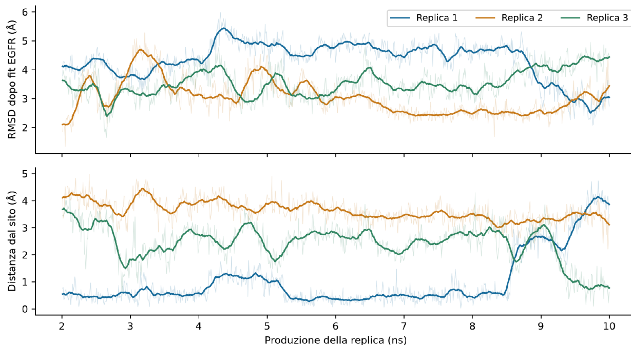
Figura 15.14B. Andamento dell'RMSD del ligando dopo fit globale di EGFR (sopra) e della distanza tra il centro del ligando e il centro del sito definito dalla geometria iniziale (sotto). Sono mostrati i frame analizzati fra 2,01 e 10 ns. Le linee sottili riportano i valori per frame; le linee marcate sono medie mobili centrate su 20 frame, pari a circa 0,2 ns, con finestre ridotte ai margini. Lo smoothing facilita la lettura e non entra nel calcolo delle statistiche.
