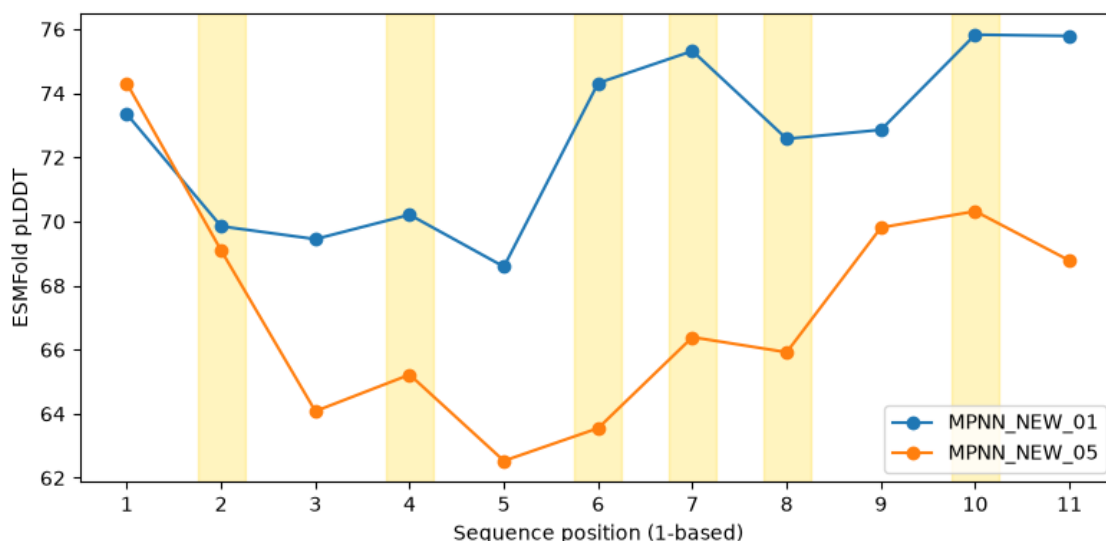
Figura 13.7a – Confidenza ESMFold nelle singole posizioni delle sequenze MPNN_NEW_01 e MPNN_NEW_05. L'asse orizzontale riporta le 11 posizioni del peptide, mentre l'asse verticale mostra il valore pLDDT assegnato da ESMFold a ciascun residuo. Valori più alti indicano una maggiore confidenza del modello nella geometria locale prevista. La linea blu rappresenta MPNN_NEW_01 e la linea arancione MPNN_NEW_05. Le bande gialle identificano le sei posizioni 2, 4, 6, 7, 8 e 10, mantenute fisse durante la progettazione con ProteinMPNN.
