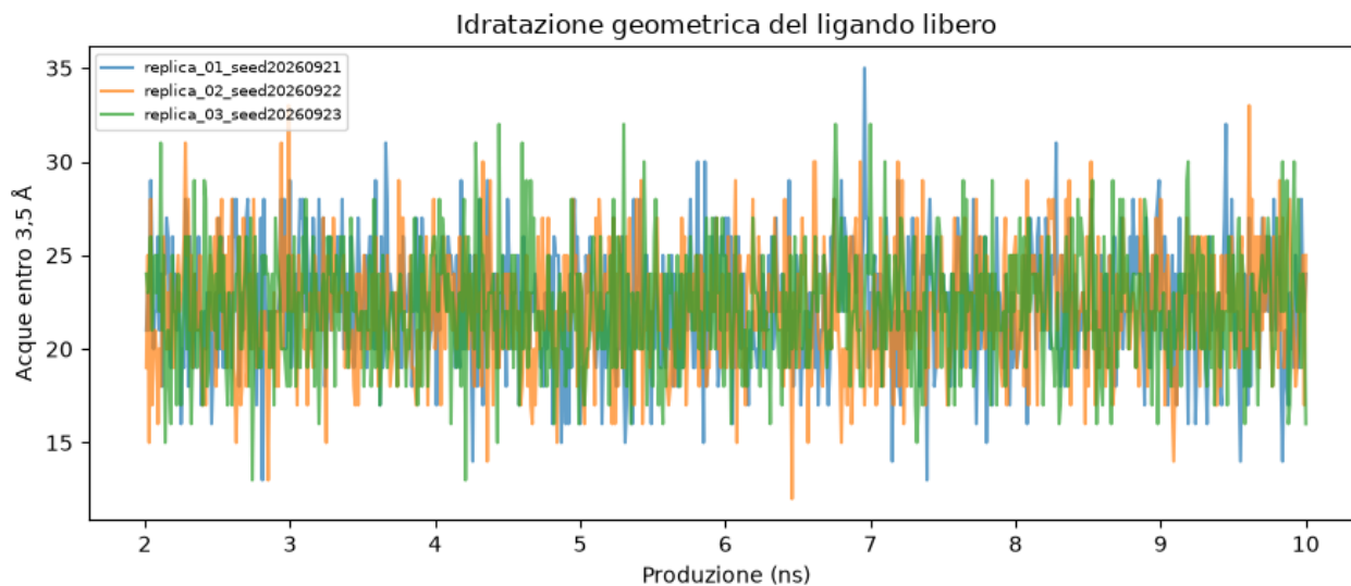
Figura 15.13B. Idratazione geometrica di MOL00583 libera in acqua nelle tre repliche 09j. È riportato, dopo lo scarto iniziale, il numero di molecole d'acqua il cui ossigeno si trova entro 3,5 Å da almeno un atomo pesante del ligando. Le tracce mostrano fluttuazioni ampiamente sovrapposte senza una deriva evidente a vista. La misura non identifica legami a idrogeno e non quantifica energia di solvatazione o tempi di residenza delle acque.
