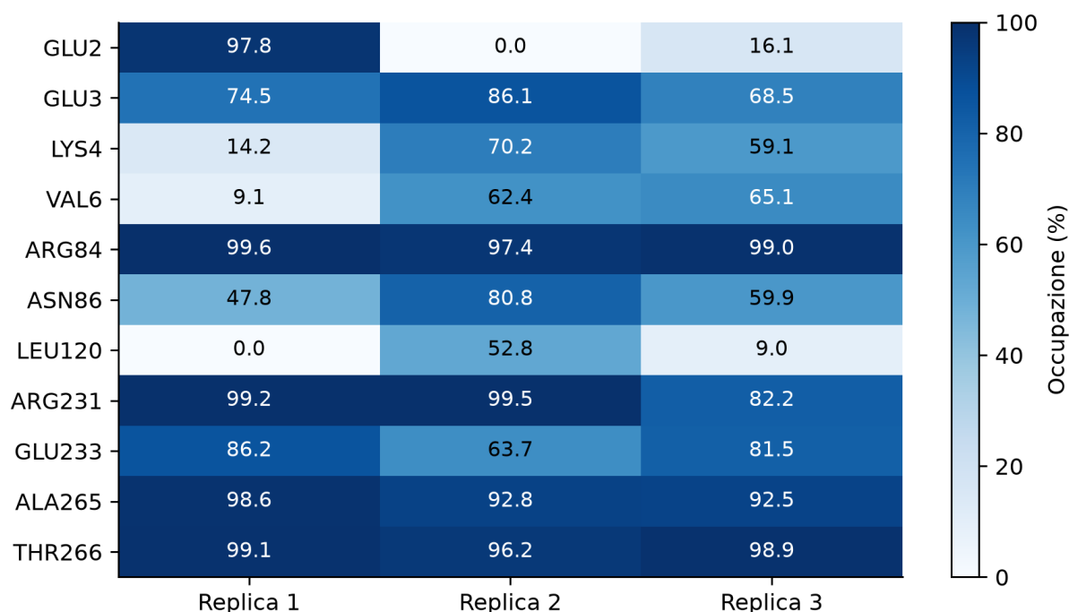
Figura 15.11C. Occupazione percentuale dei contatti ligando–EGFR nelle tre repliche 09k, dopo lo scarto iniziale. Sono inclusi i residui che raggiungono almeno il 50% in una replica; sono riportati anche i valori inferiori alla soglia nelle altre repliche. I contatti sono definiti dalla distanza minima tra atomi pesanti inferiore a 4 Å. Non equivalgono necessariamente a legami a idrogeno né a contributi energetici favorevoli.
