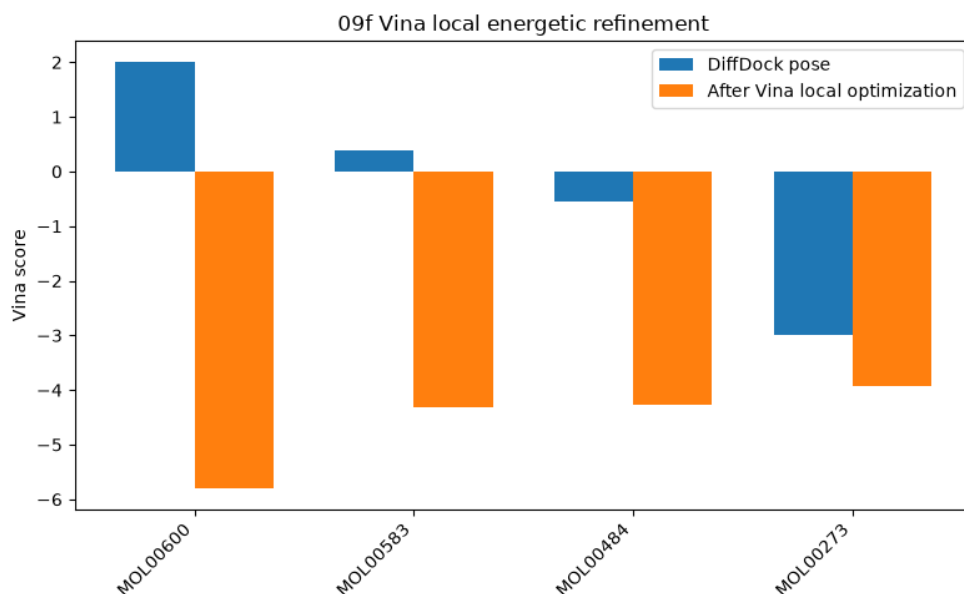
Figura 15.6 – Confronto tra lo score Vina della posa DiffDock iniziale e quello ottenuto dopo l'ottimizzazione locale. Valori più negativi indicano una valutazione relativamente più favorevole secondo la funzione di scoring di Vina. MOL00600 raggiunge lo score finale migliore, ma richiede anche la correzione energetica più ampia rispetto alla posa iniziale.
