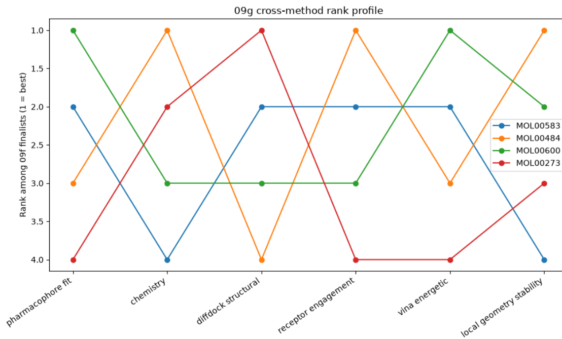
Figura 15.7B – Ranking storico dei quattro finalisti nei sei assi di valutazione utilizzati da 09g. Il rank 1 indica il risultato più favorevole e il rank 4 quello meno favorevole all'interno del gruppo. La figura documenta il criterio multi-dominio che ha determinato la selezione originaria di MOL00583, ma i sei assi non rappresentano sei evidenze indipendenti né costituiscono un ranking specifico per la native EGF–EGFR interface. Le successive verifiche site-specifiche mostrano infatti che la posa di MOL00583 propagata nel follow-up è off-site, mentre MOL00484 conserva supporto strutturale pertinente all'interfaccia EGF.
