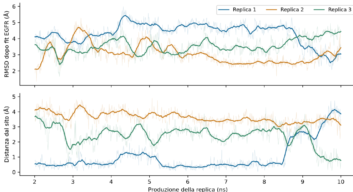
Figura 15.11B. Andamento dell'RMSD del ligando dopo fit globale di EGFR (sopra) e della distanza tra il centro del ligando e il centro del sito definito dalla geometria iniziale (sotto). Sono mostrati i frame analizzati fra 2,01 e 10 ns. Le linee sottili riportano i valori per frame; le linee marcate sono medie mobili centrate su 20 frame, pari a circa 0,2 ns, con finestre ridotte ai margini. Lo smoothing facilita la lettura e non entra nel calcolo delle statistiche.
