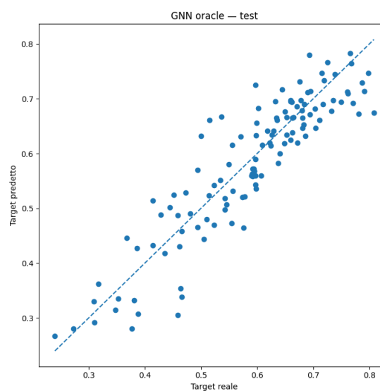
Figura 7.4f — Oracle GNN: target predetto e target computazionale di riferimento nel test set.
