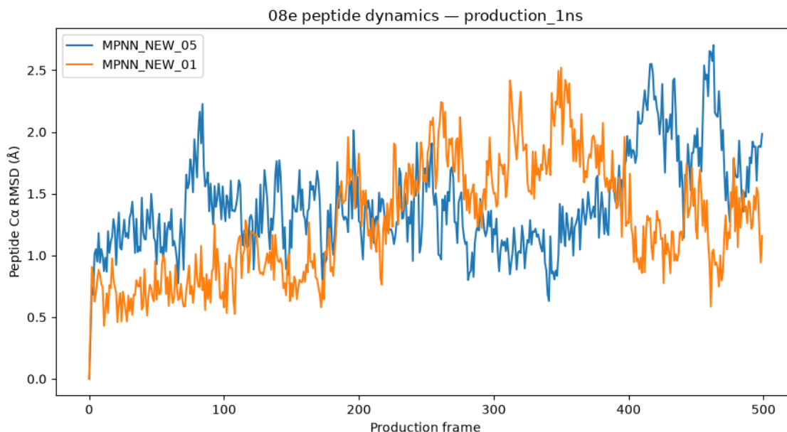
Figura 13.5a – Andamento dell'RMSD dei due peptidi ProteinMPNN durante la simulazione di produzione. Le curve mostrano la deviazione degli atomi Ca di MPNN_NEW_01 e MPNN_NEW_05 rispetto alla conformazione iniziale, dopo l'allineamento del recettore. L'asse orizzontale riporta i 500 frame salvati durante 1 ns di produzione, mentre l'asse verticale esprime l'RMSD in ångström. Valori più bassi indicano una minore deviazione dalla conformazione iniziale. Sono rappresentati soltanto i due nuovi candidati perché il notebook 08e esegue nuove simulazioni MD esclusivamente per MPNN_NEW_01 e MPNN_NEW_05.
