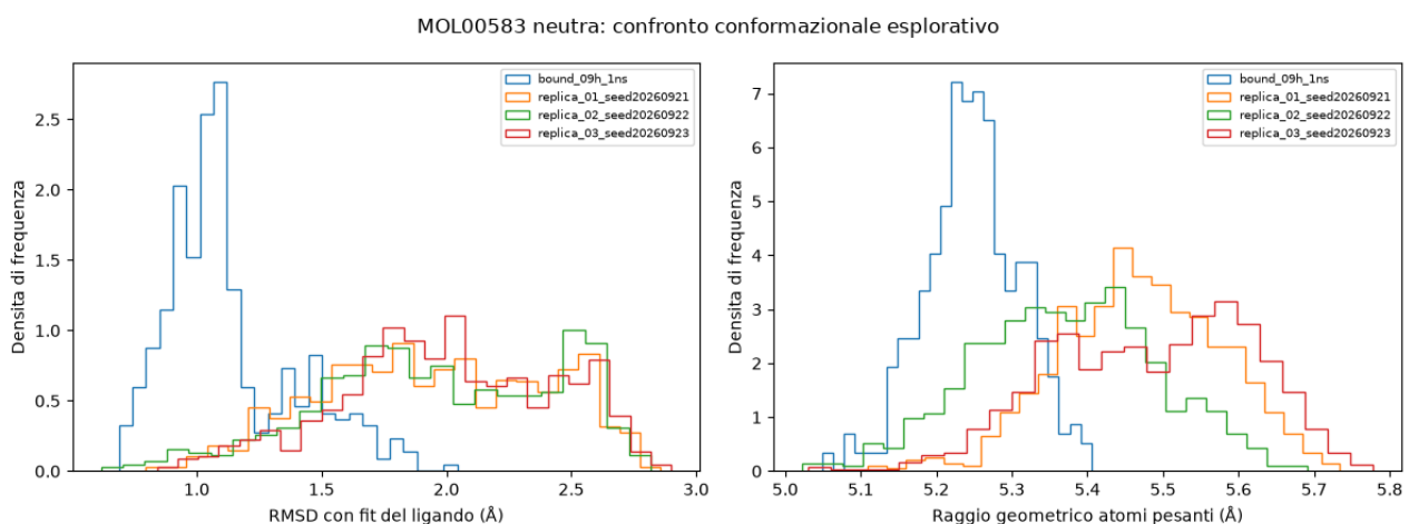
Figura 15.10. Confronto preliminare tra MOL00583 libera in acqua (tre repliche 09j da 10 ns) e nel complesso della simulazione 09h da 1 ns. A sinistra, distribuzione dell'RMSD con fit del ligando rispetto a 09f; a destra, raggio geometrico degli atomi pesanti. È escluso il primo 20% di ciascuna produzione. Le finestre di campionamento differiscono: gli istogrammi descrivono le traiettorie disponibili e non costituiscono un test di significatività o di convergenza.
