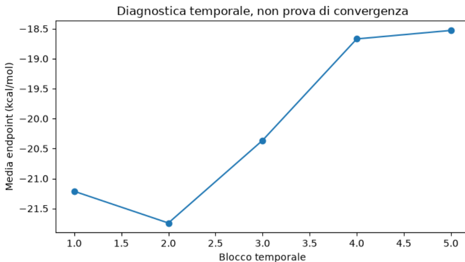
Figura 15.12. Variazione temporale del proxy energetico endpoint di MOL00583-EGFR. I 50 snapshot analizzati nell'intervallo 202–1.000 ps sono suddivisi in cinque blocchi temporali consecutivi di 10 snapshot ciascuno. Le energie medie risultano rispettivamente pari a -21,21 , -21,74 , -20,36 , -18,67 e -18,53 kcal/mol. Il passaggio a valori meno negativi nei blocchi finali evidenzia una variazione temporale del supporto energetico e suggerisce cautela nell'assumere convergenza. Le linee collegano le medie per facilitarne la lettura; i blocchi appartengono alla stessa traiettoria e non rappresentano repliche indipendenti. Il grafico non dimostra dissociazione né misura un'affinità sperimentale.
