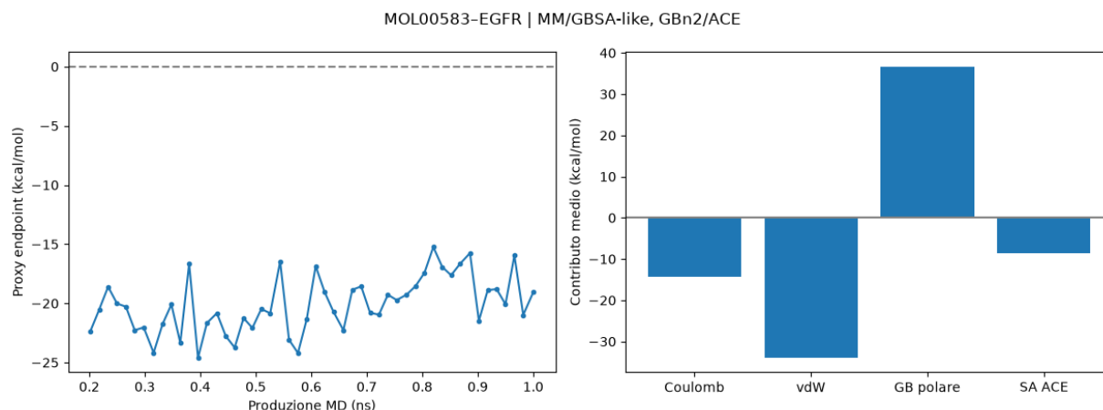
Figura 15.11. Analisi energetica endpoint del complesso MOL00583-EGFR mediante il protocollo MM/GBSA-like GBn2/ACE. A sinistra, andamento del proxy energetico su 50 snapshot distribuiti nell'intervallo 202–1.000 ps della produzione MD, dopo esclusione del primo 20% della traiettoria. A destra, contributi medi elettrostatico diretto (Coulomb), van der Waals (vdW), solvatazione polare GB e superficiale ACE. Il valore complessivo medio è -20,10 kcal/mol, con deviazione standard di 2,37 kcal/mol tra gli snapshot. Nella parte finale il proxy tende a diventare meno negativo; il risultato non dimostra pertanto convergenza raggiunta. I valori descrivono una stima endpoint senza contributo entropico e non equivalgono a un'energia libera rigorosa di binding o a un'affinità sperimentale. Gli snapshot provengono da una singola traiettoria, sono temporalmente correlati e non costituiscono repliche indipendenti.
