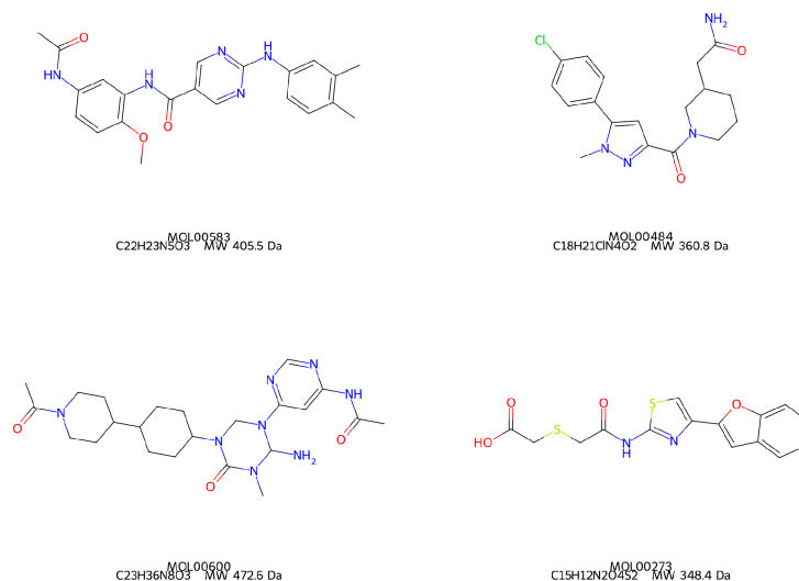
Figura 15.8 – Strutture chimiche bidimensionali dei quattro finalisti della Pipeline 5. MOL00583 è il lead computazionale primario; MOL00484, MOL00600 e MOL00273 sono mantenuti come alternative ortogonali. Tutti provengono dalla rescue track.
