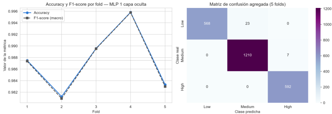
Figura 10. Accuracy y F1-score macro por fold (izquierda) y matriz de confusión agregada de los 5 folds (derecha) — modelo campeón, K-Fold estratificado k=5.
