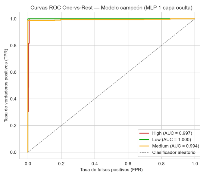
Figura 11. Curvas ROC One-vs-Rest del modelo campeón (MLP 1 capa oculta) sobre el conjunto de prueba.
