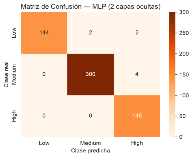
Figura 8. Matriz de confusión del modelo MLP 2 capas ocultas sobre el conjunto de prueba.
