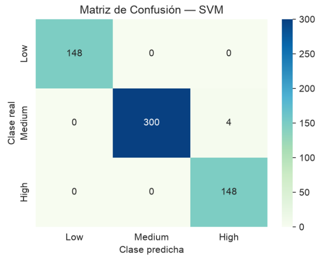
Figura 5. Matriz de confusión del modelo SVM sobre el conjunto de prueba.
