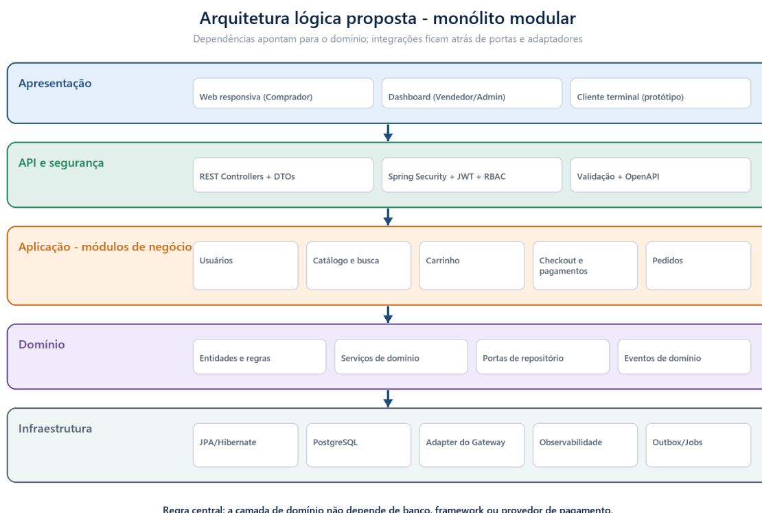
Figura 9.1 - Arquitetura lógica em camadas e módulos.
