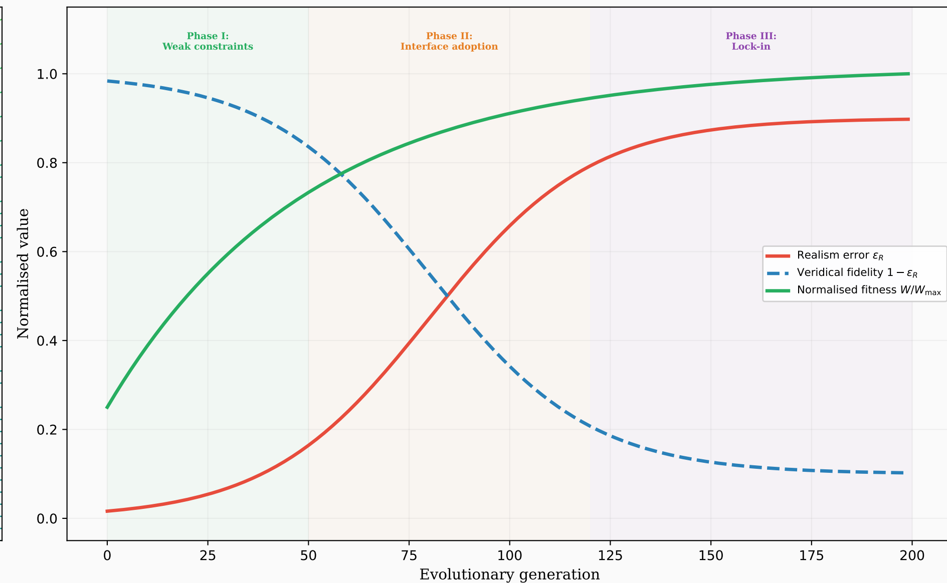
(d) Evolutionary Trajectory: Realism \rightarrow Interface Lock-in
