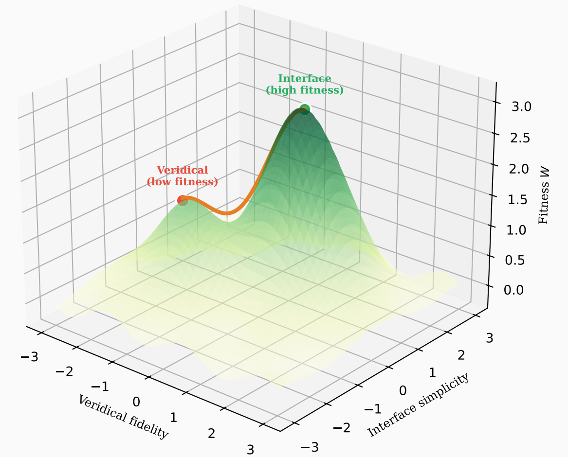
(d) Evolutionary Trajectory: Realism \rightarrow Interface Lock-in
