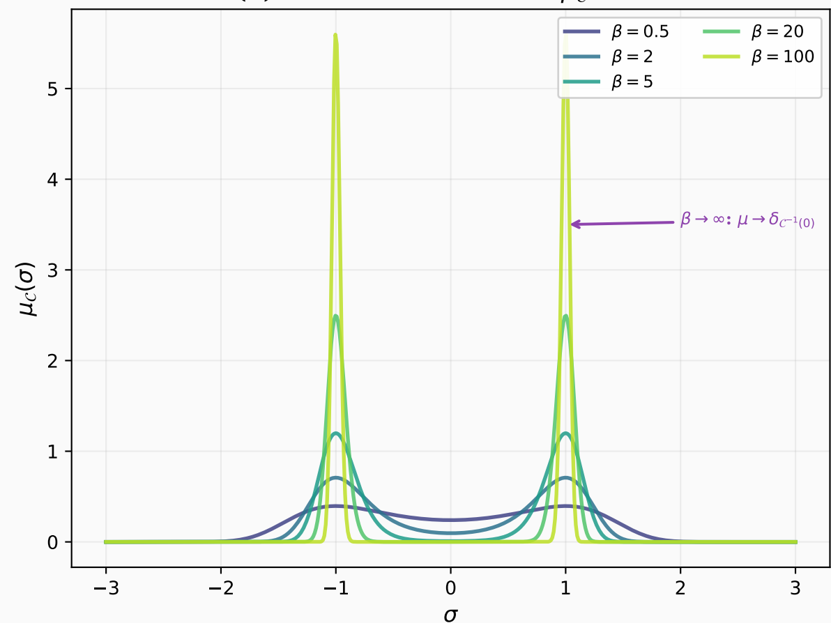
(d) Microcanonical Entropy
