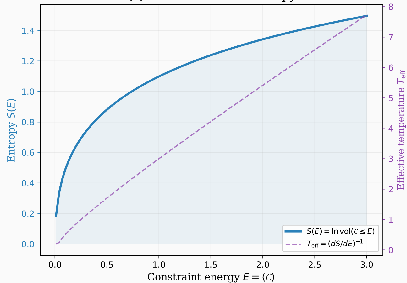
(d) Microcanonical Entropy
