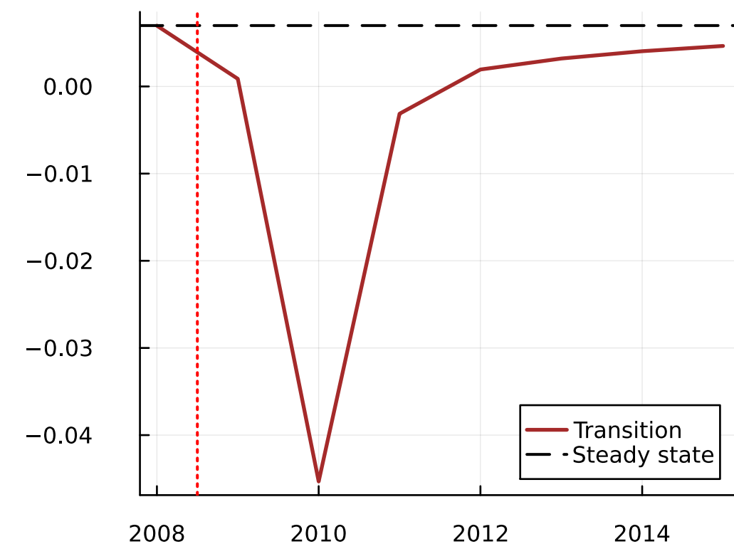
r_t
