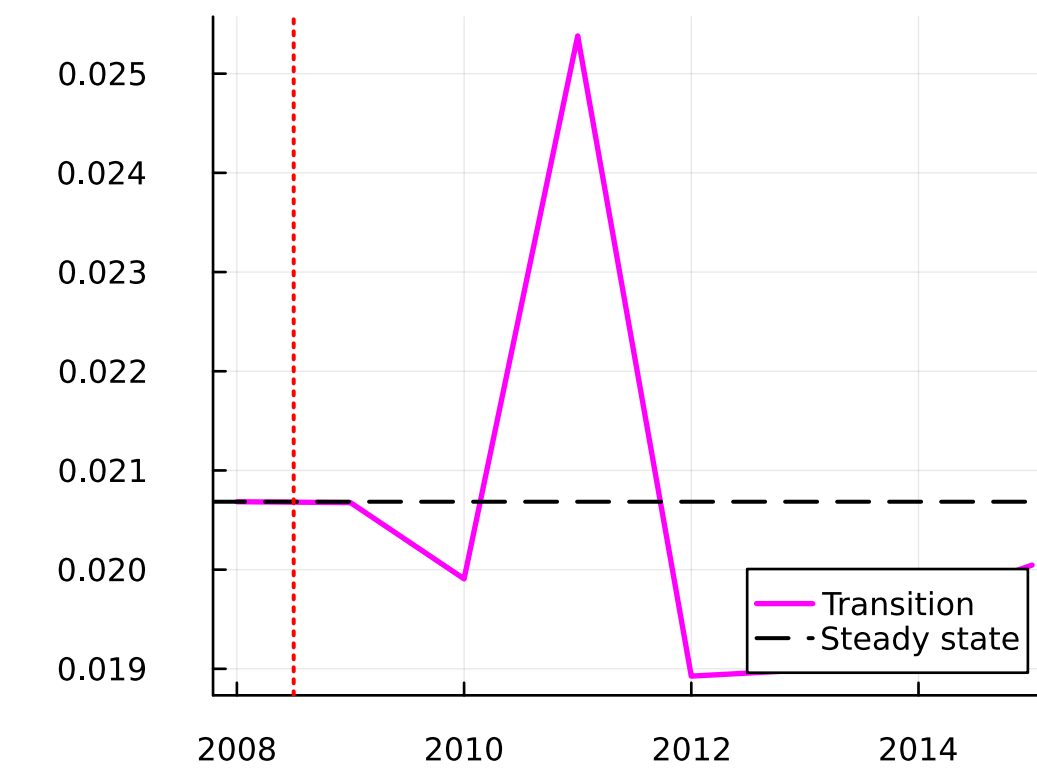
\mathbb{E}[o(z,a)=1]
