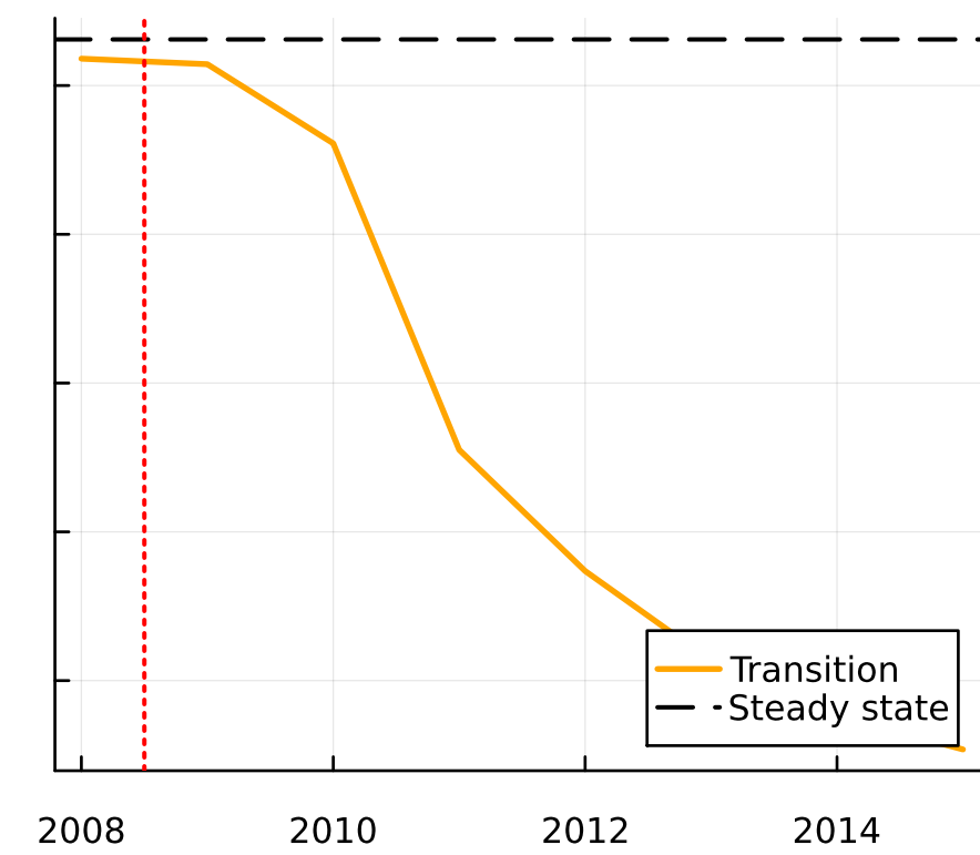
r_t
